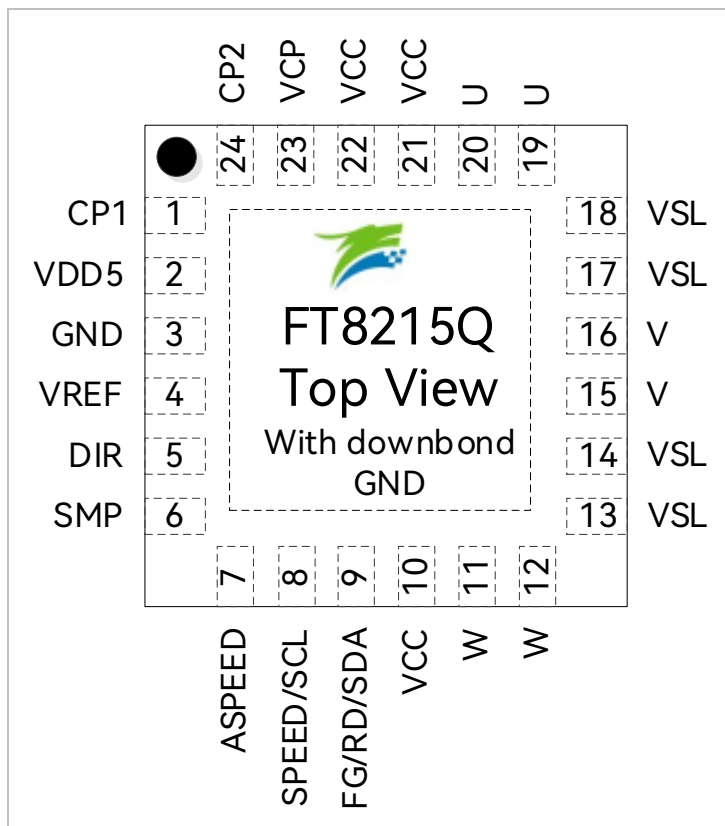
图 1-6 FT8215Q QFN24 引脚图
