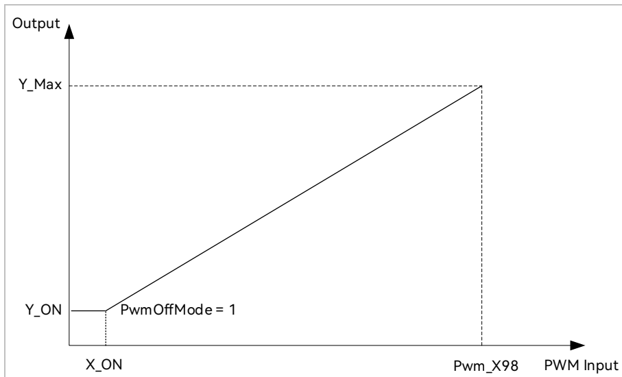
图 5-4 速度环或电流环模式下的曲线 (PwmOffMode = 1)
