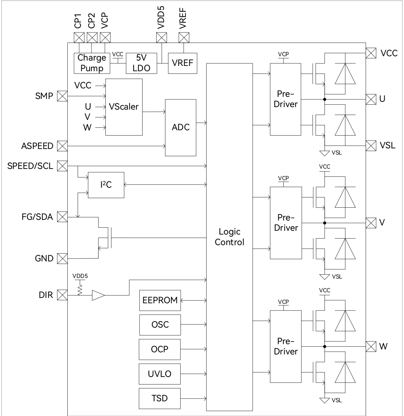
图 1-5 FT8215Q / FT8215P 功能框图
