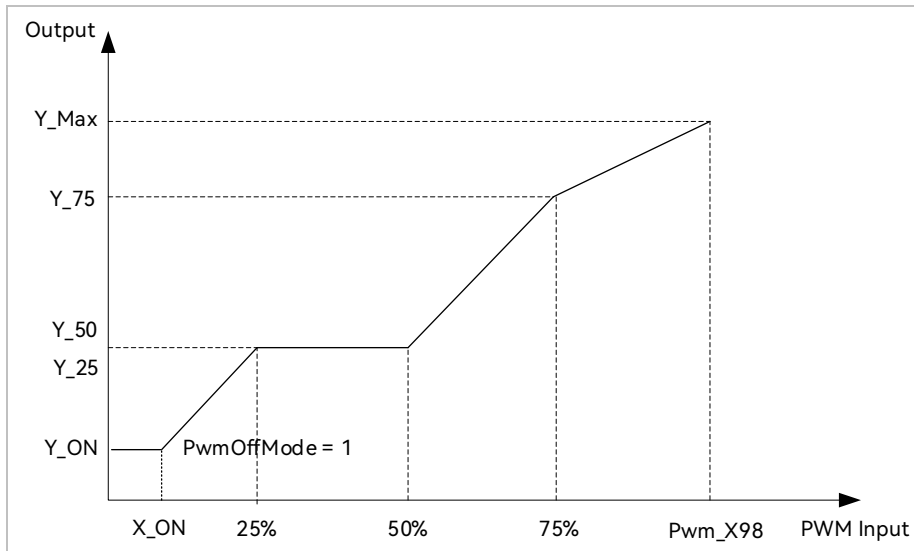
图 5-2 电压环模式下的曲线 (PwmOffMode = 1)
