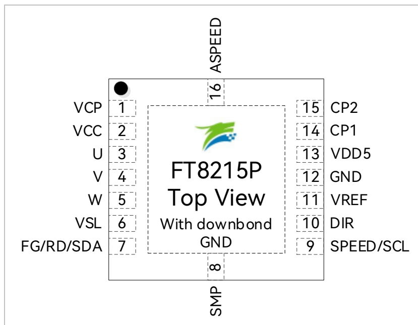
图 1-7 FT8215P PLQFN16 引脚图
