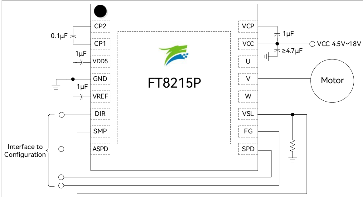
图 1-4 FT8215P 应用电路（双电阻/三电阻）
