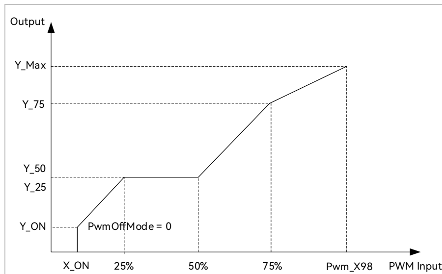
图 5-1 电压环模式下的曲线 (PwmOffMode = 0)
