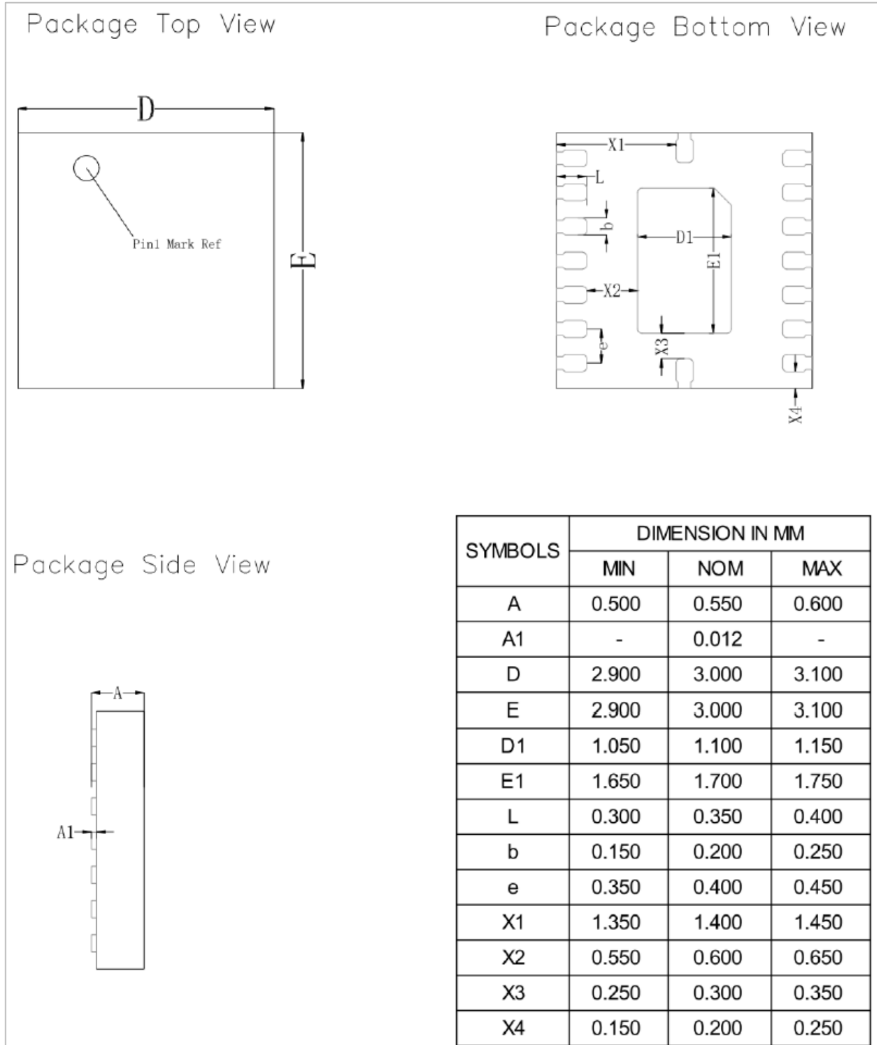
图 2-2 FT8215P PLQFN16_3X3 封装尺寸图
