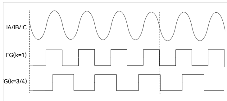
图 5-7 k = 1 和 k = 3/4 的 FG 输出图
