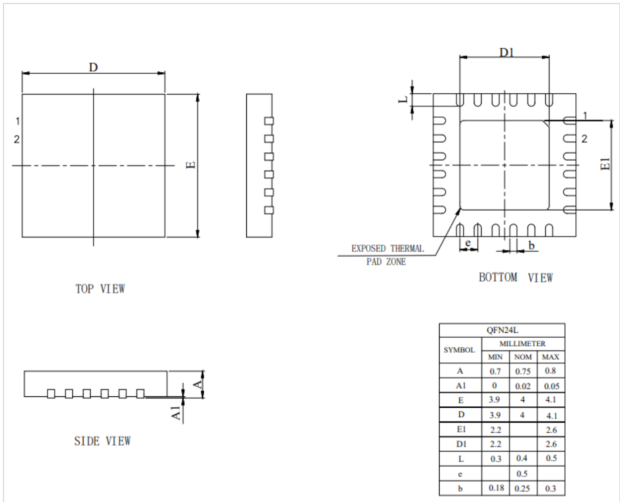
图 2-1 FT8215Q QFN24_4X4 封装尺寸图
