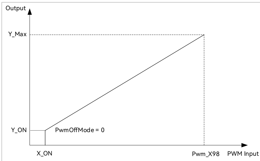
图 5-3 速度环或电流环模式下的曲线 (PwmOffMode = 0)
