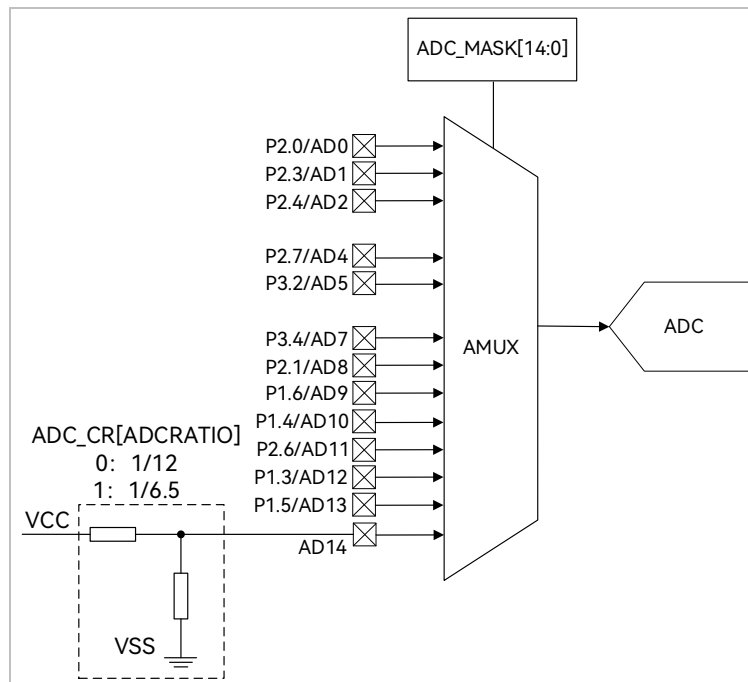
图 22-1 ADC 多路复用器框图
