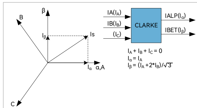
图 12-3 Clarke 变换
