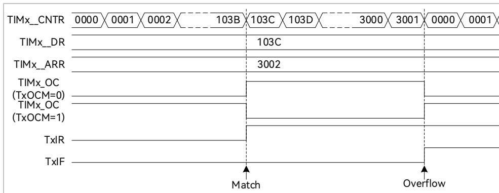
图 15-2 输出模式输出波形
