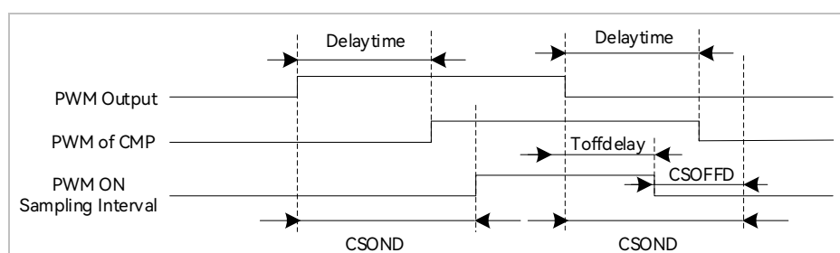
图 28-13 PWM ON 采样模式
