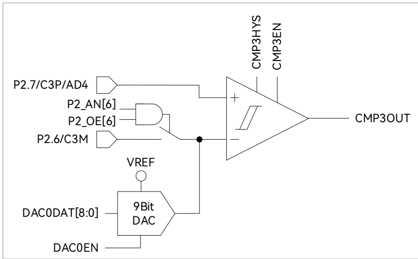
图 28-3 双比较器输入模式
