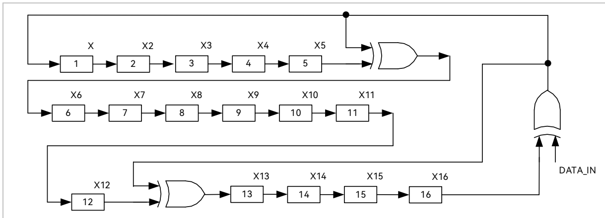
图 31-2 CRC16 电路原理图
