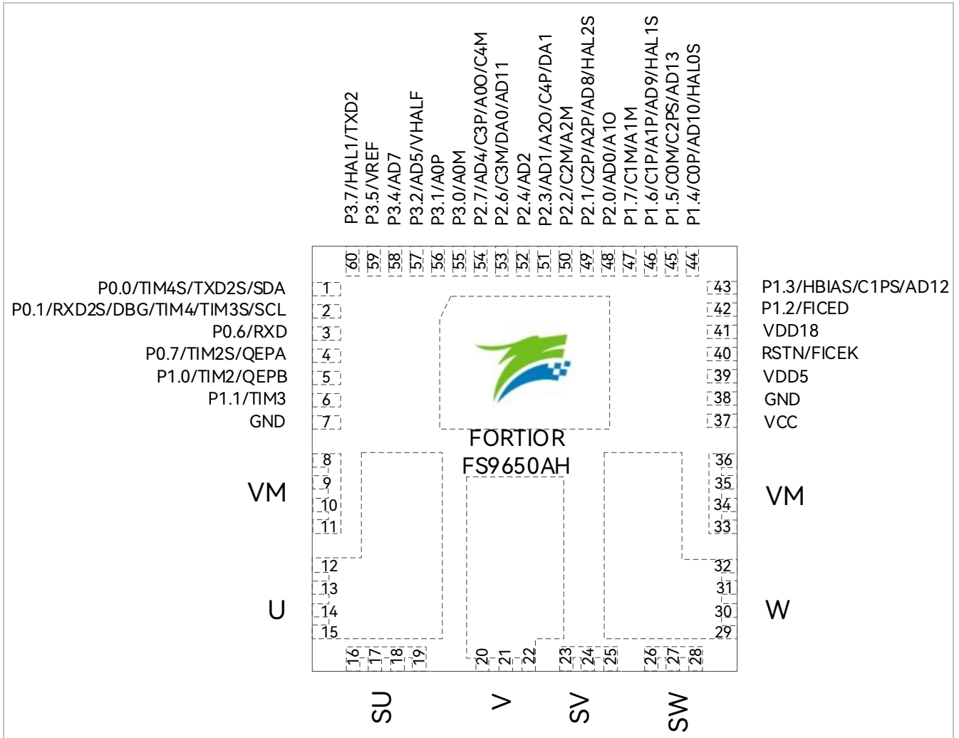
图 2-1 FS9650AH QHF8080-60L 引脚图
