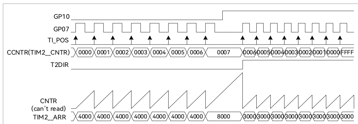
图 14-13 步进模式时序图
