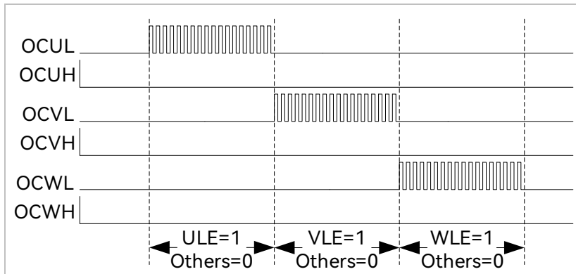
图 17-6 刹车波形图
