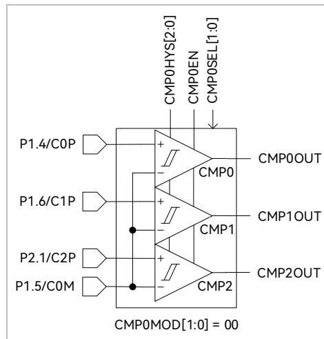
图 28-8 无内置电阻三比较器模式
