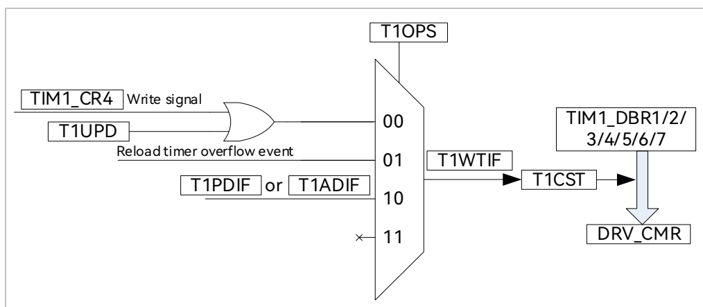
图 13-9 写入时序框图
