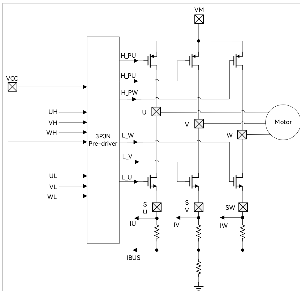
图 17-1 Pre-driver 模块框图
