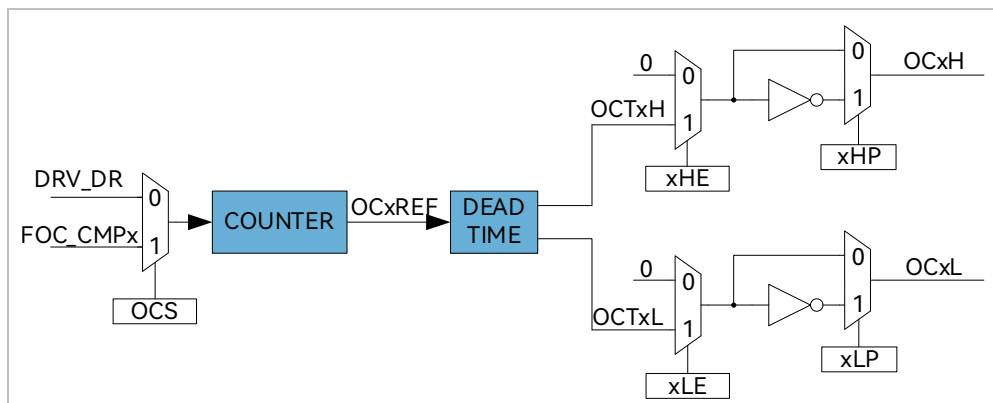
图 17-2 输出控制模块前级框图
