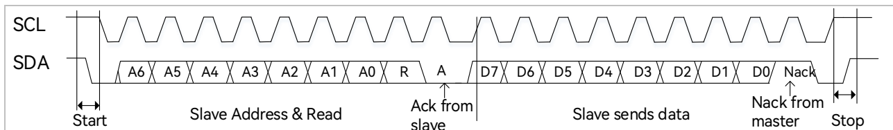
图 8-3 主机接收从机的数据
