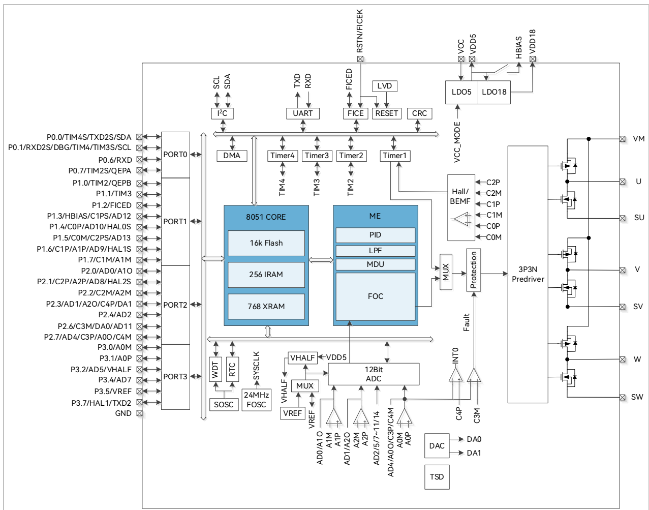
图 1-1 FS9650AH 功能框图
