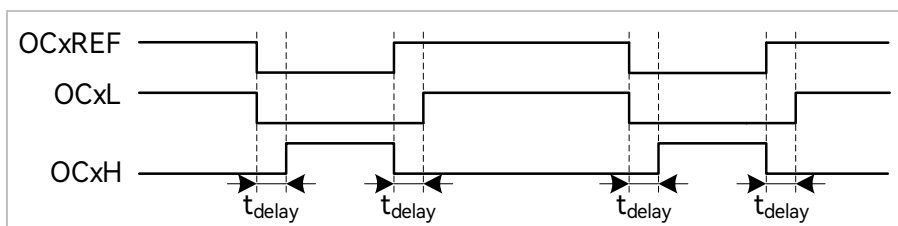
图 17-4 带死区插入的互补输出
