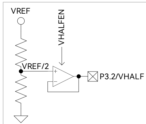
图 26-1 VHALF 模块输入输出端口
