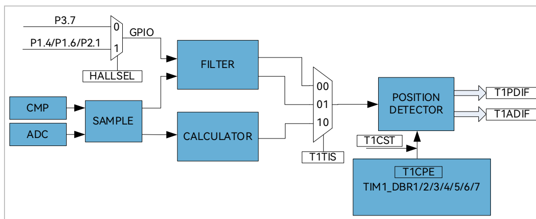
图 13-5 位置检测功能框图
