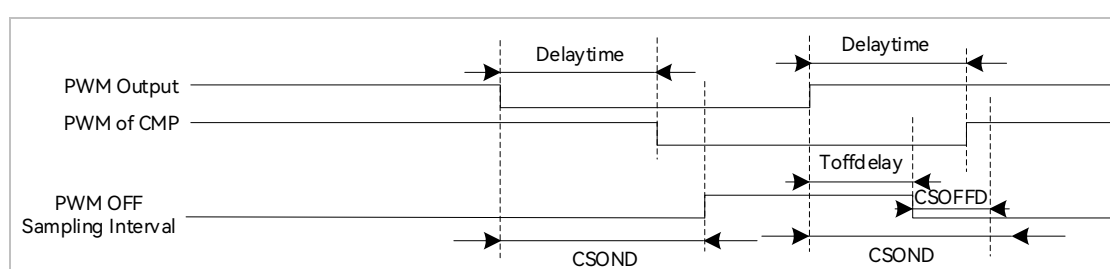
图 28-14 PWM OFF 采样模式
