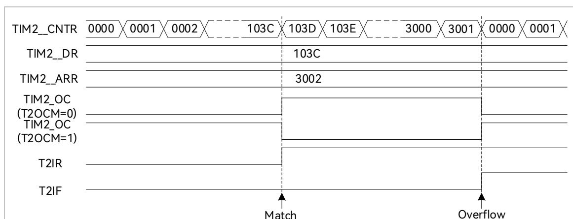
图 14-2 输出模式输出波形
