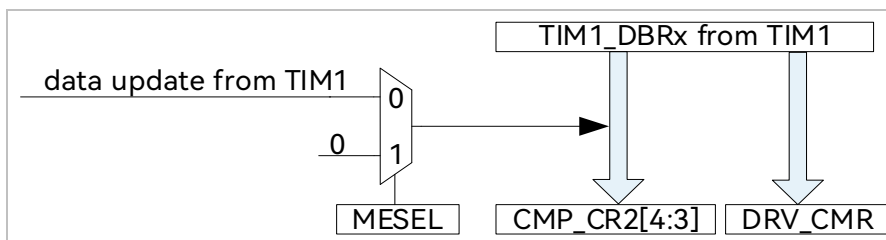
图 17-7 Timer1 自动控制 DRV_CMx 和 CMP_CR2[4:3]
