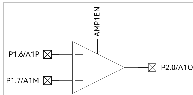
图 27-4 AMP1 输入输出相关端口
