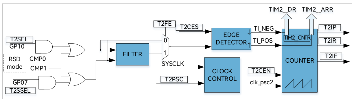
图 14-5 输入捕获模式原理框图
