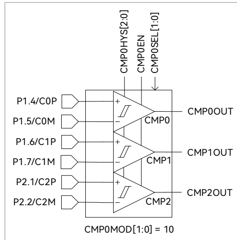
图 28-11 三差分比较器模式
