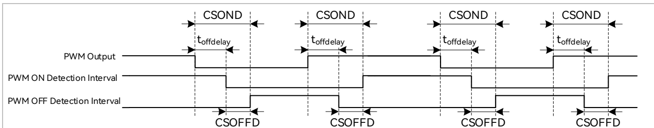
图 13-7 采样区间图
