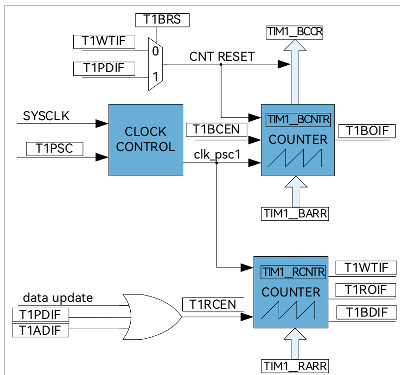
图 13-2 时基单元
