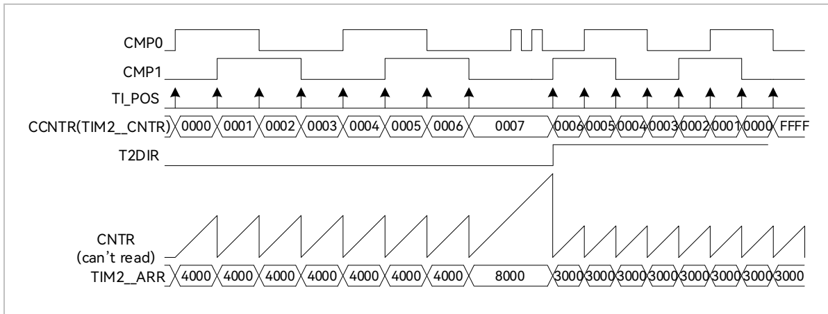
图 14-10 QEP&RSD 模式时序图
