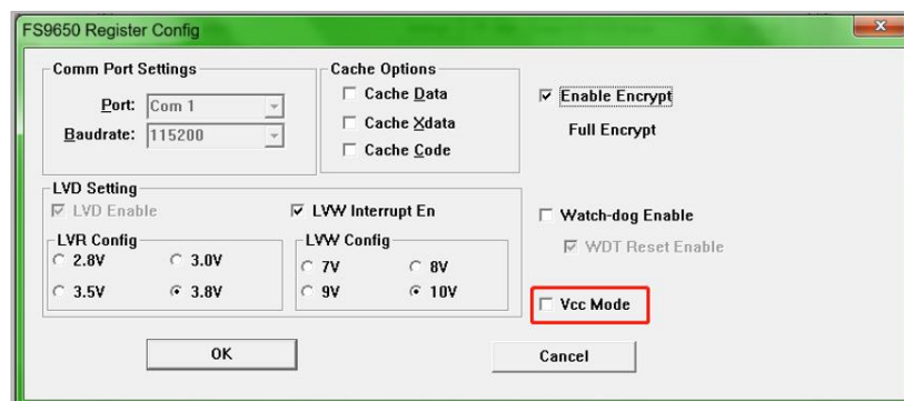
图 29-2 VCC_MODE 配置
