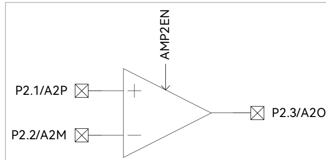
图 27-5 AMP2 输入输出相关端口
