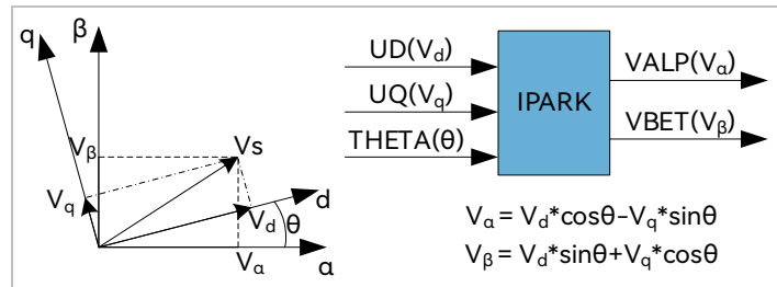
图 12-2 Park 逆变换
