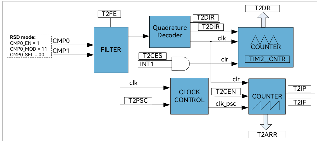
图 14-9 RSD 模式原理框图
