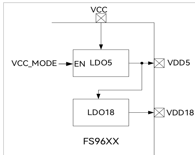
图 29-1 电源模块功能框图
