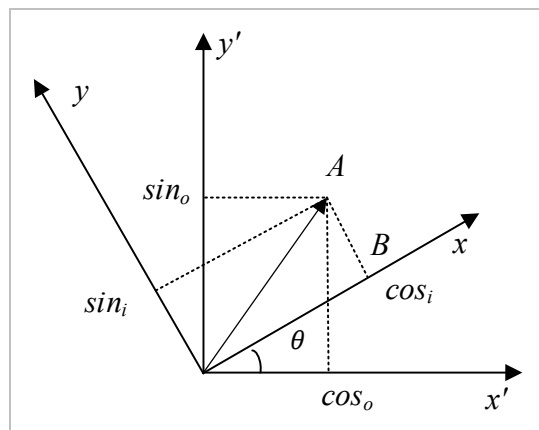
图 10-1 坐标变换
