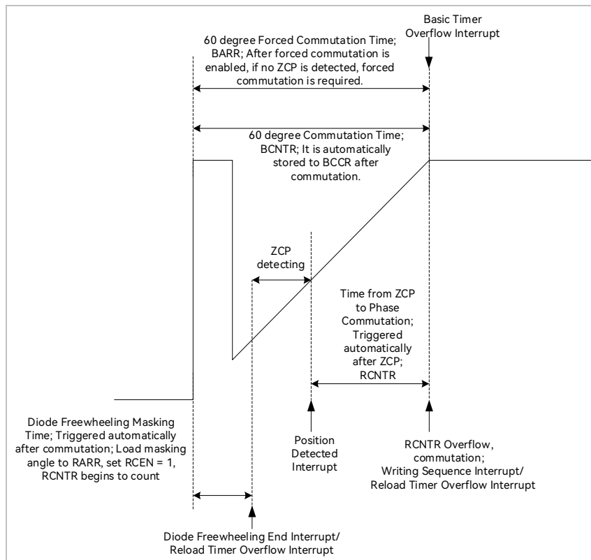
图 13-12 BLDC 的工作原理
