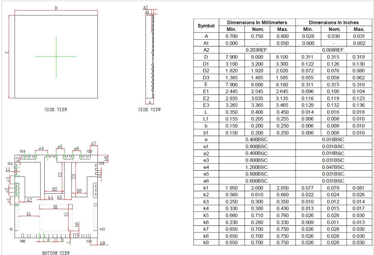
图 3-1 FS9650AH QHFBP8080-60L_8x8 封装尺寸图
