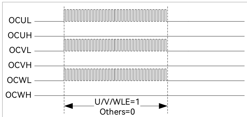
图 17-6 刹车波形图
