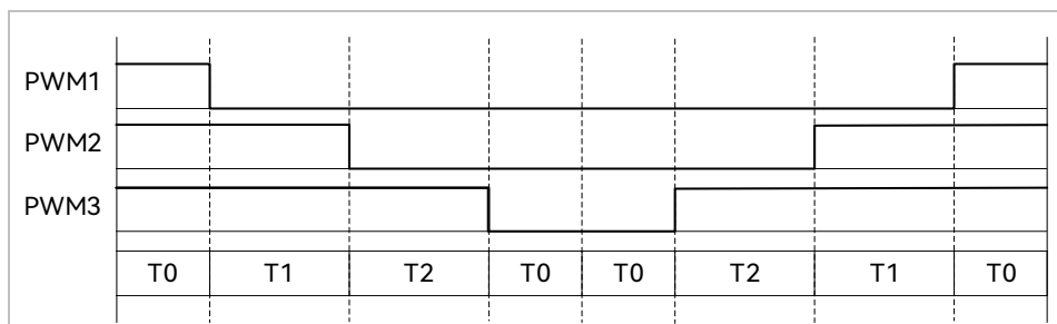
图 12-7 七段式 SVPWM 输出电平
