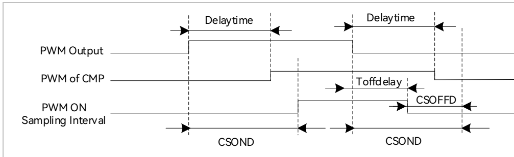
图 14-11 PWM ON 采样模式
