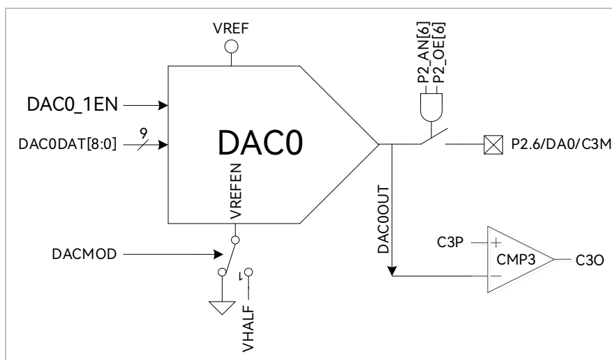
图 23-1 DAC0 功能框图
