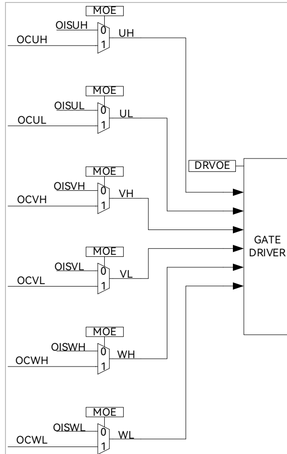
图 17-8 输出控制模块后级框图
