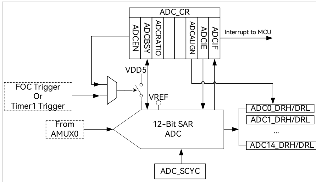
图 22-2 ADC 功能框图
