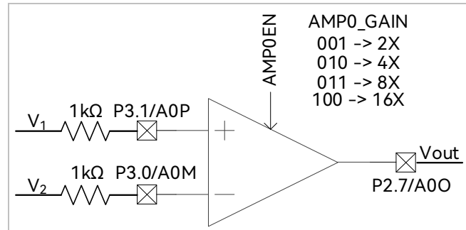
图 27-3 AMP0 工作在 PGA 差分输入模式
