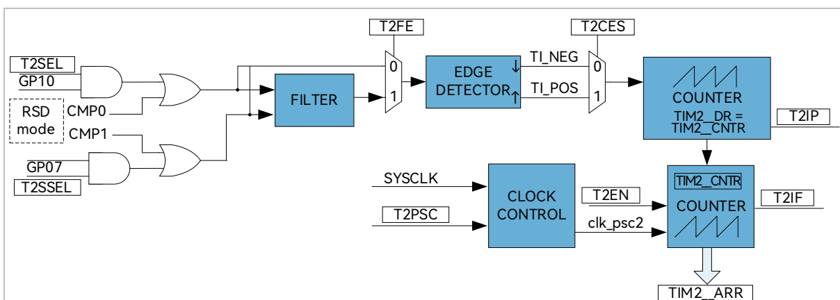
图 14-7 输入计数模式原理框图
