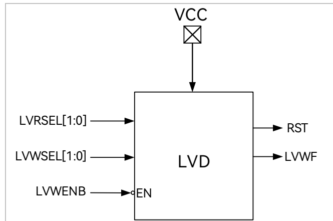
图 29-3 低电压检测模块
