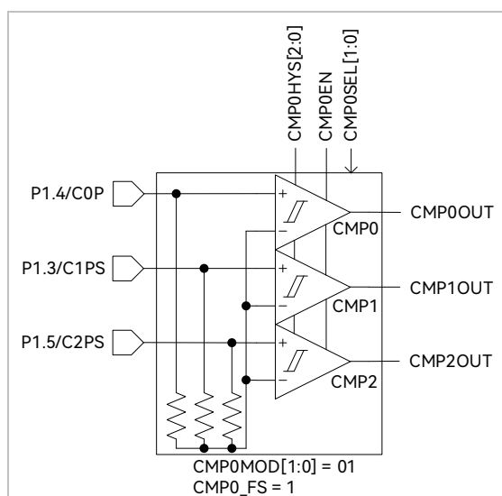
图 28-10 有内置电阻三比较器模式，功能转移
