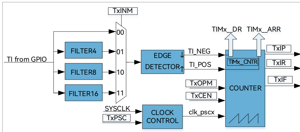
图 15-5 输入捕获模式原理框图
