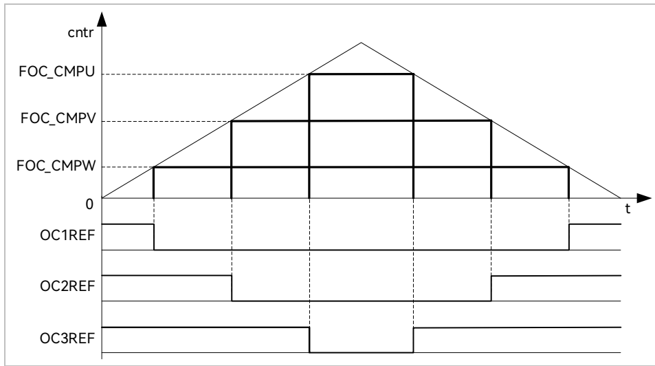
图 17-3 PWM 生成图
