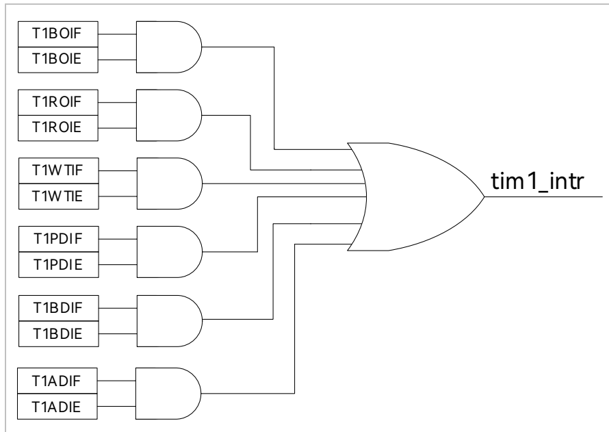
图 13-10 Timer1 中断源
