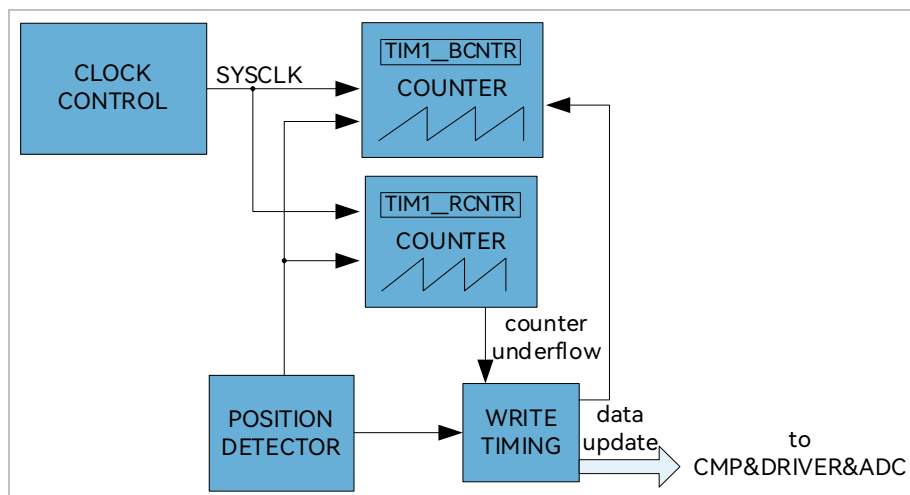
图 13-1 Timer1 内部结构
