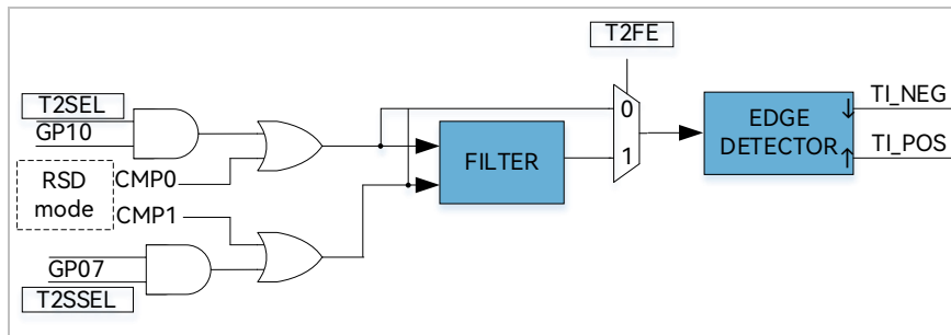
图 14-3 输入信号滤波和边沿检测框图
