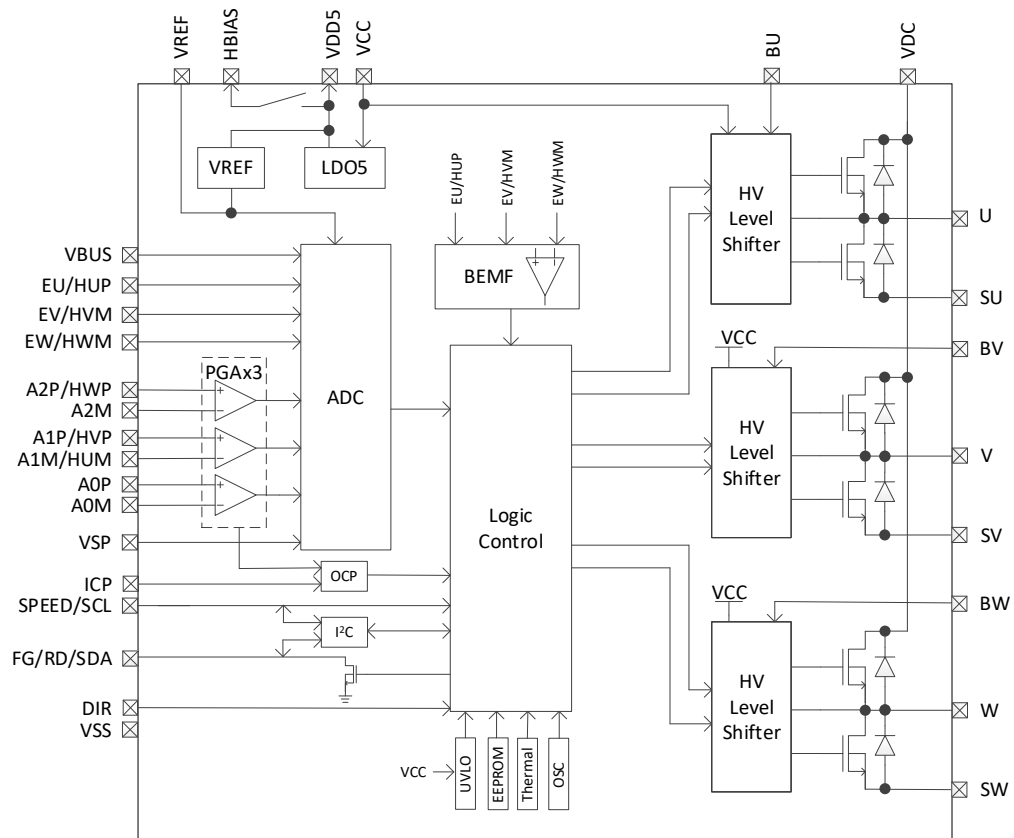
图 1-6 FS9236AS 功能框图
