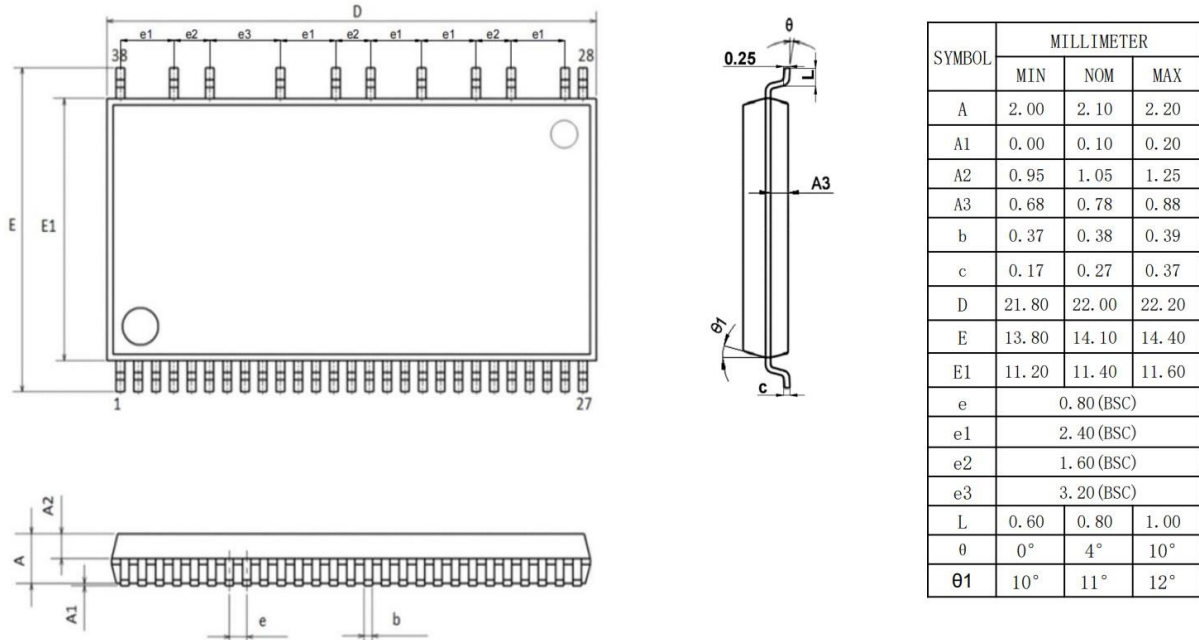
图 2-1 FS9236AS SSOP A54-38 封装尺寸图
