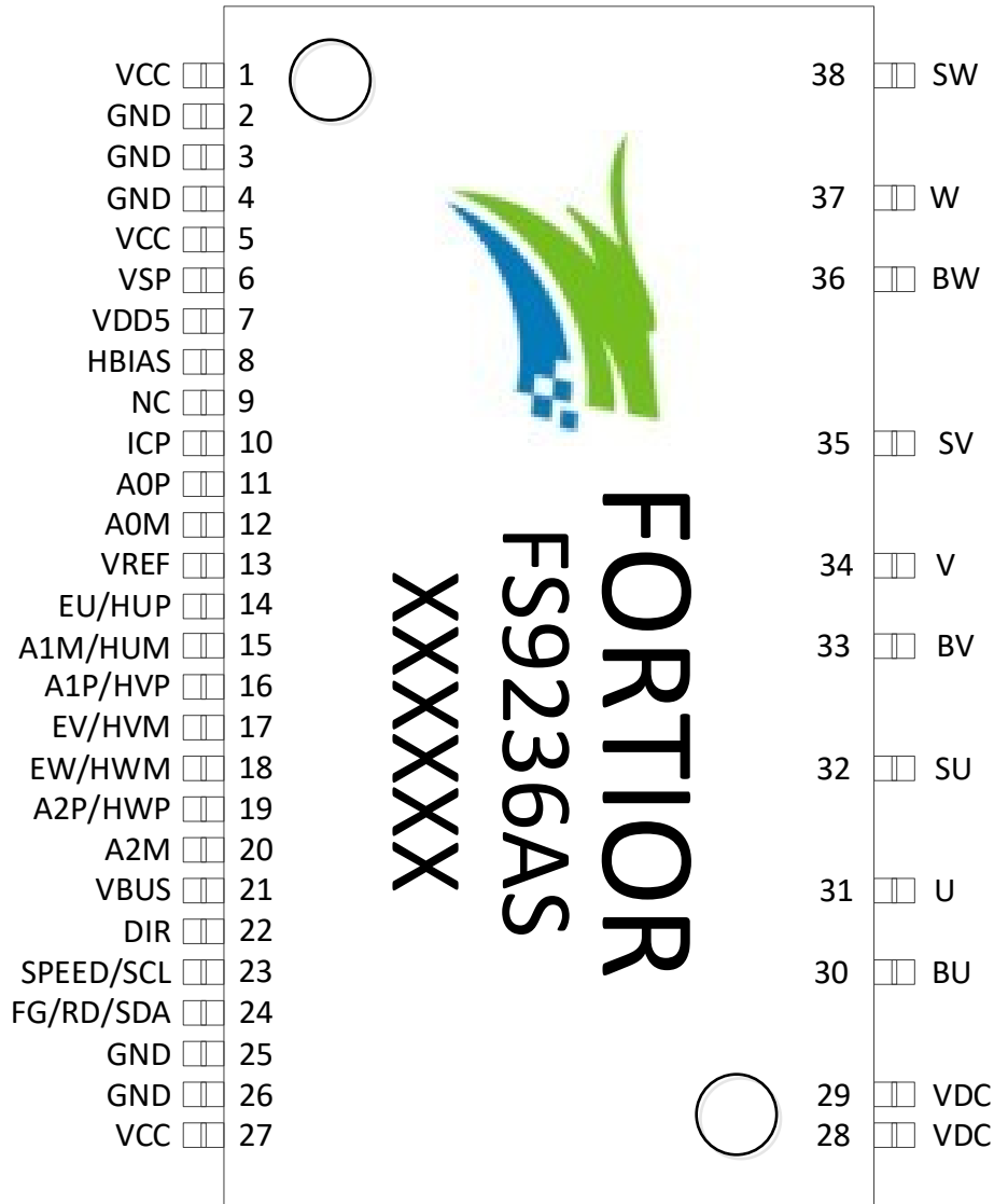
图 1-7 FS9236AS SSOP A54-38 引脚图
