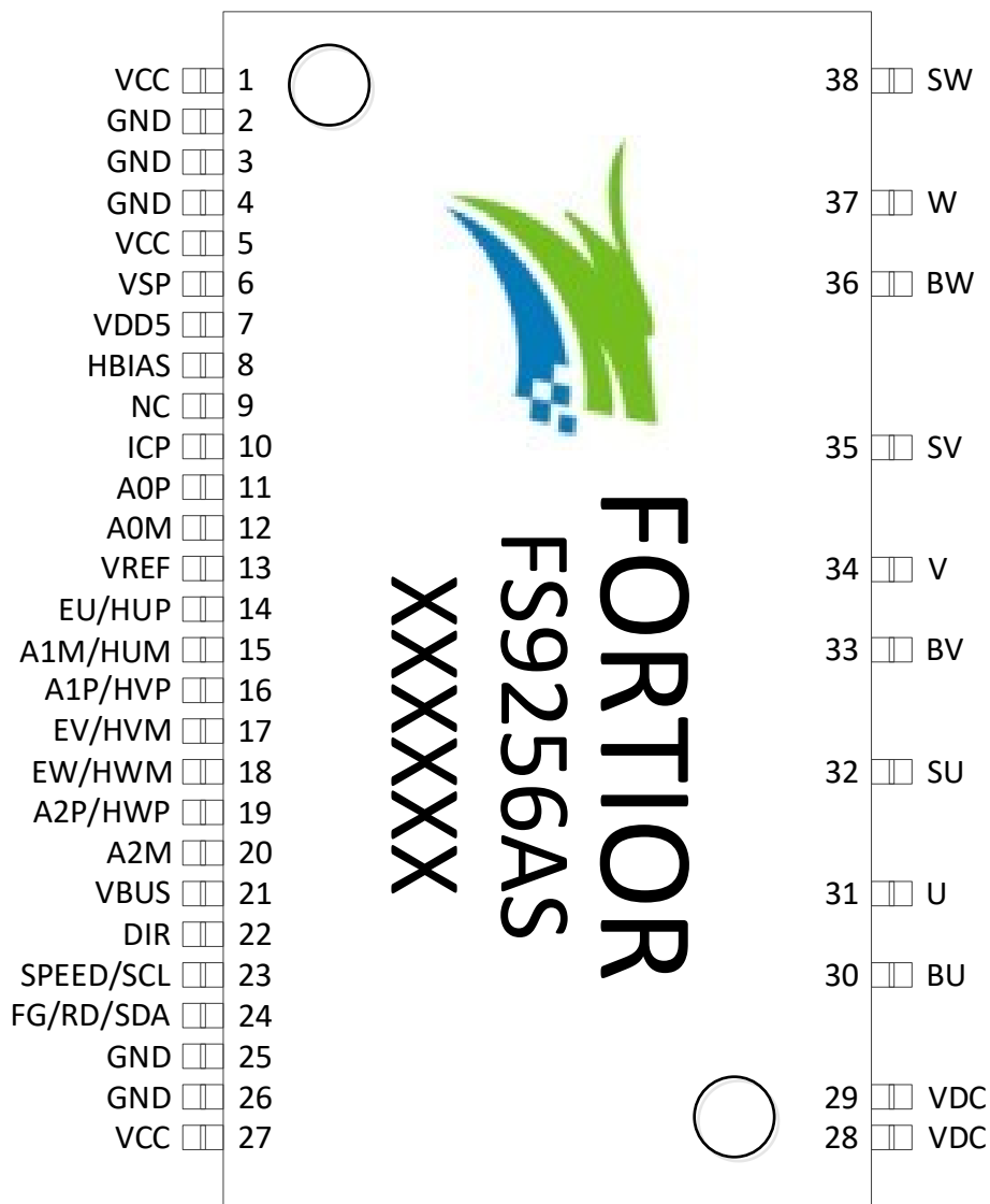
图 1-7 FS9256AS SSOP A54-38 引脚图
