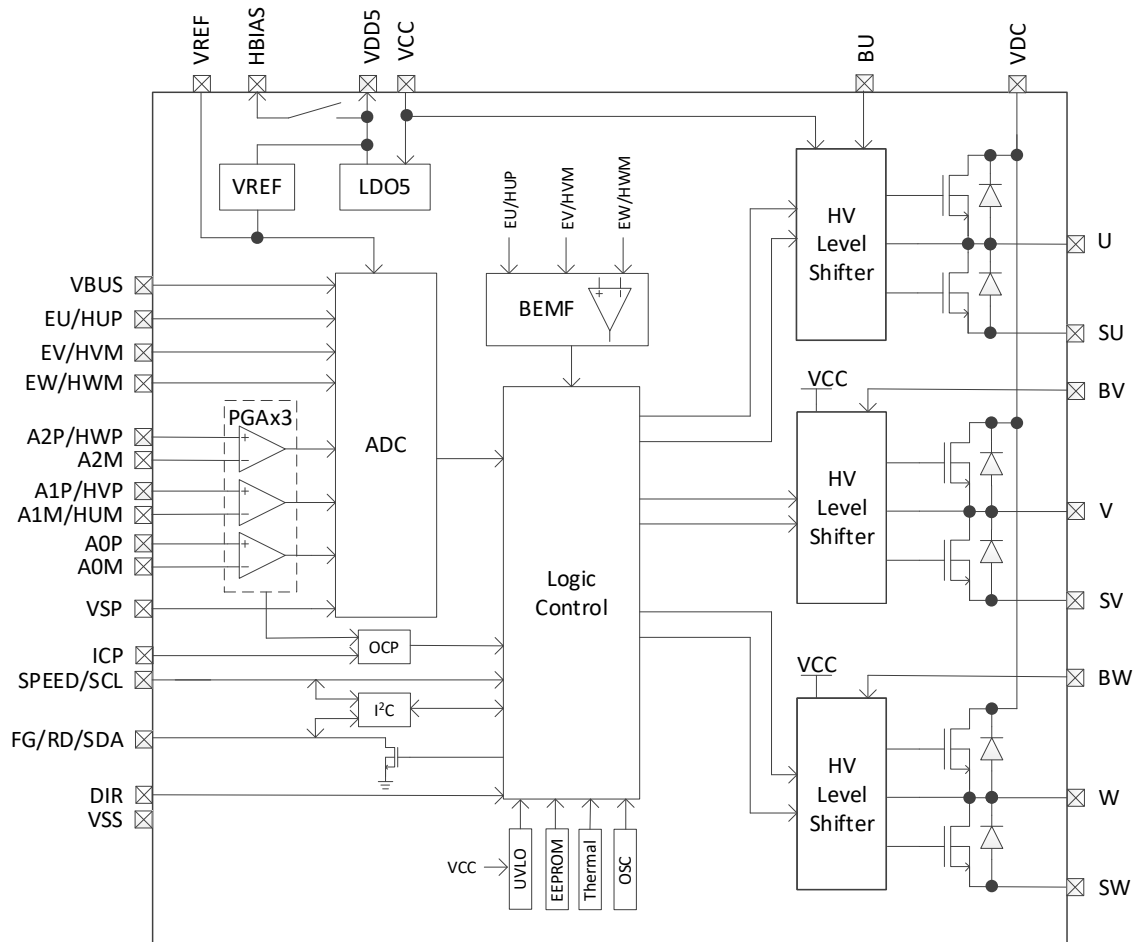
图 1-6 FS9256AS 功能框图
