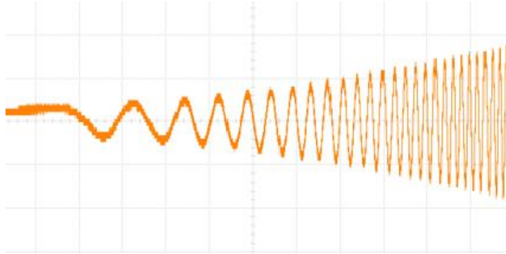
图 5-5 Soft-On 相电流波形
