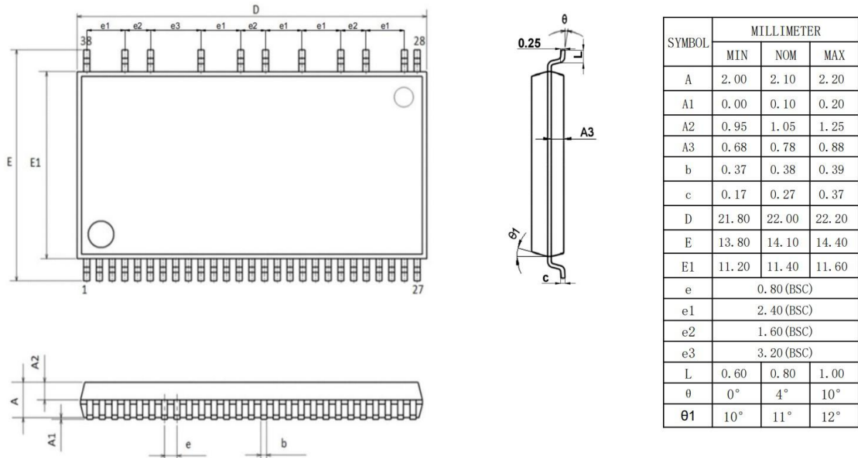
图 2-1 FS9256AS SSOP A54-38 封装尺寸图
