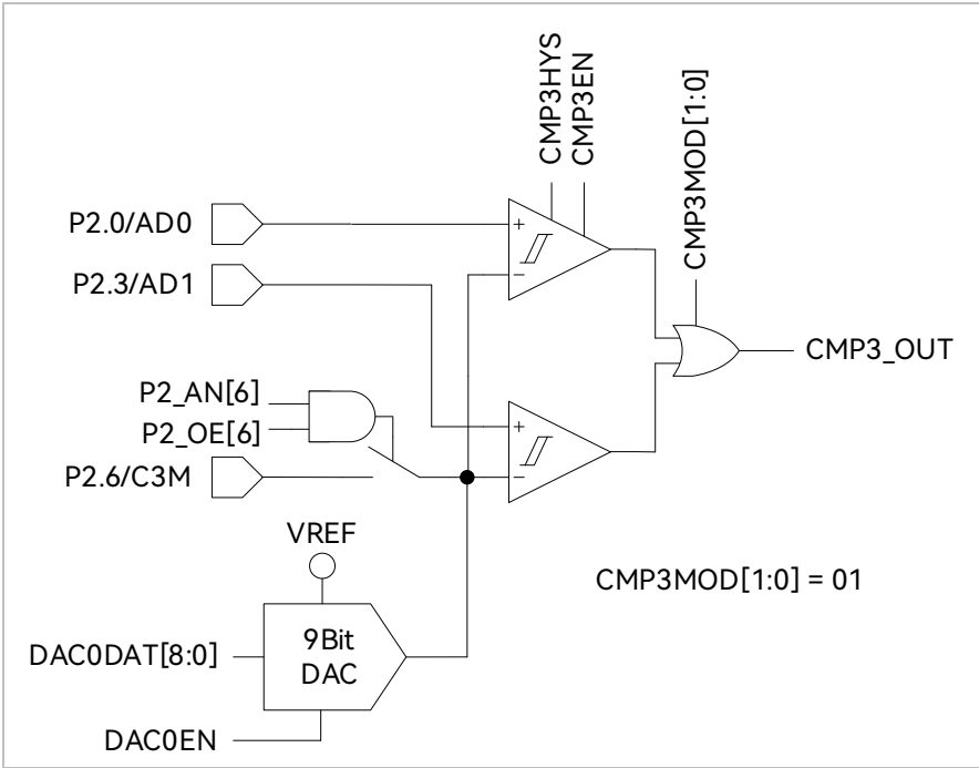
图 31-3 双比较器输入模式 (FU6867Q 不支持此模式)
