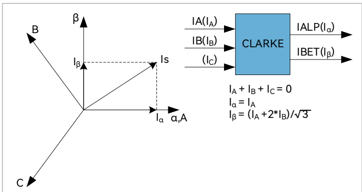
图 14-3 Clarke 变换
