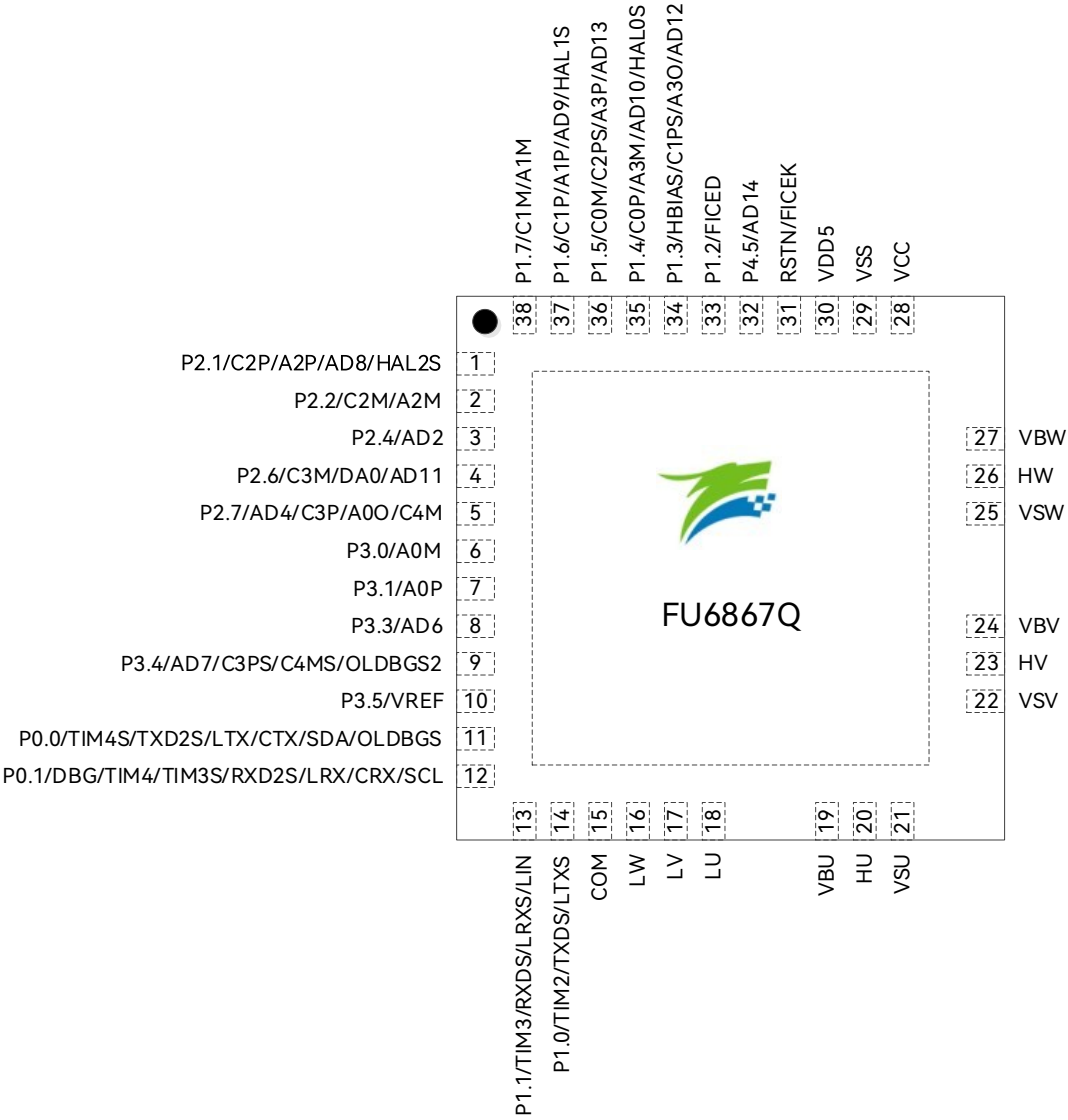
图 2-3 FU6867Q QFN48-38 引脚图
