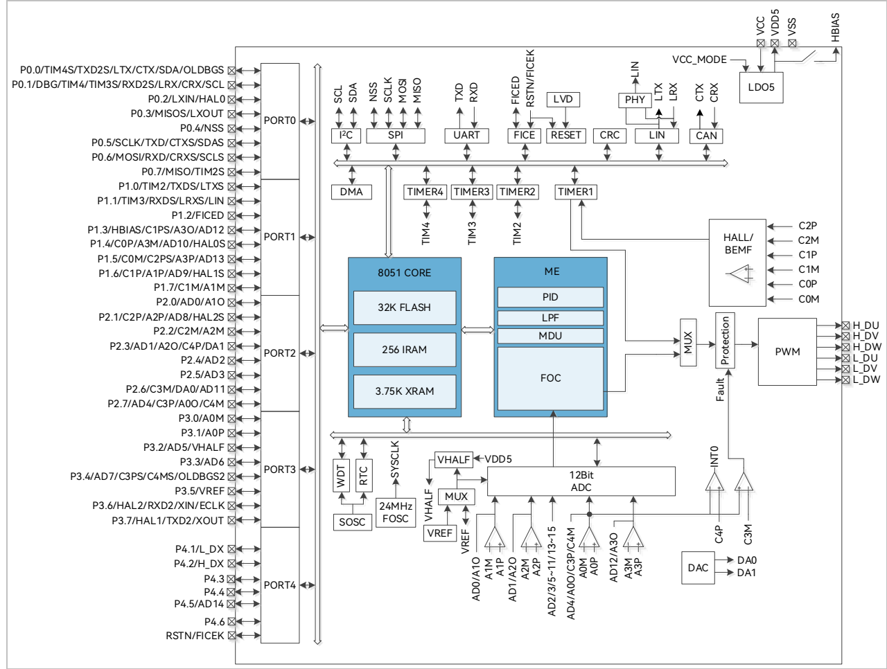
图 1-1 FU6816L 功能框图
