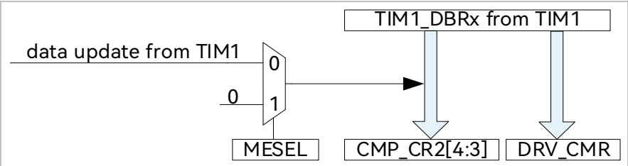
图 19-8 Timer1 自动控制 DRV_CM[R 和 CMP_CR2[4:3]
