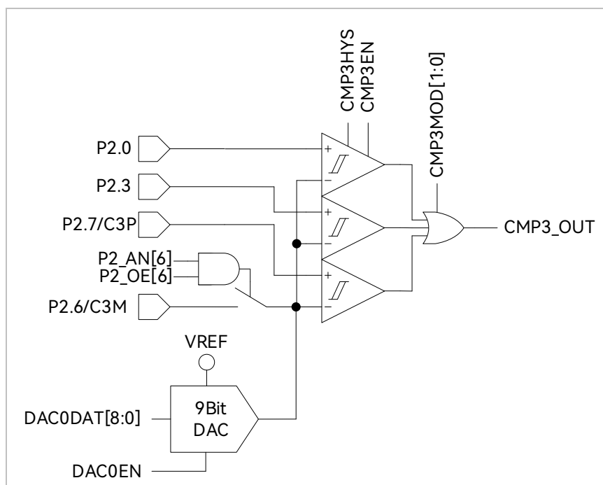
图 31-4 三比较器输入模式 (FU6867Q 不支持此模式)
