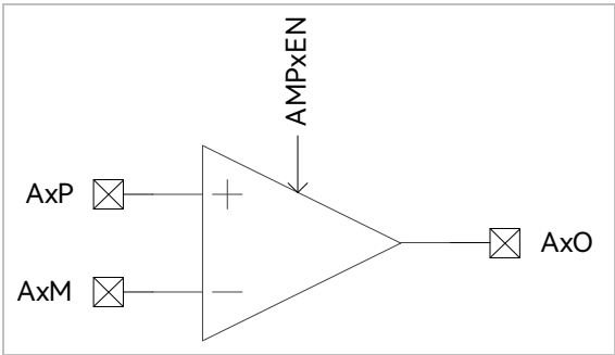
图 30-1 运算放大模块示意图
