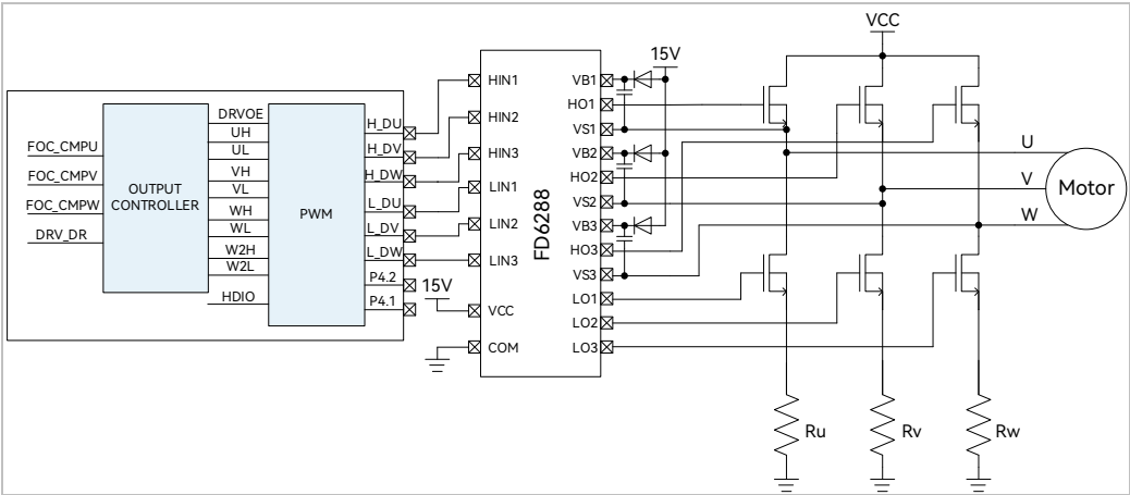
图 19-1 FU6816L Driver 模块框图
