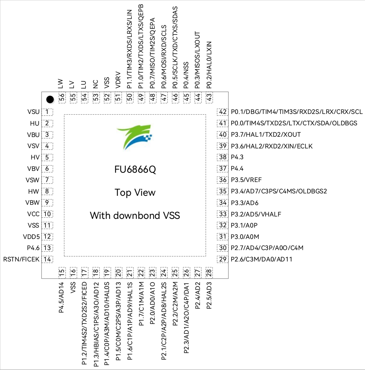
图 2-2 FU6866Q QFN56 引脚图
