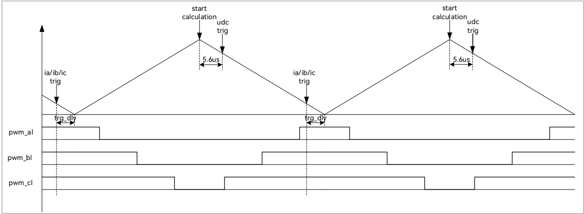
图 14-12 双三电阻电流交替采样模式
