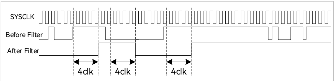
图 17-4 滤波模块时序图
