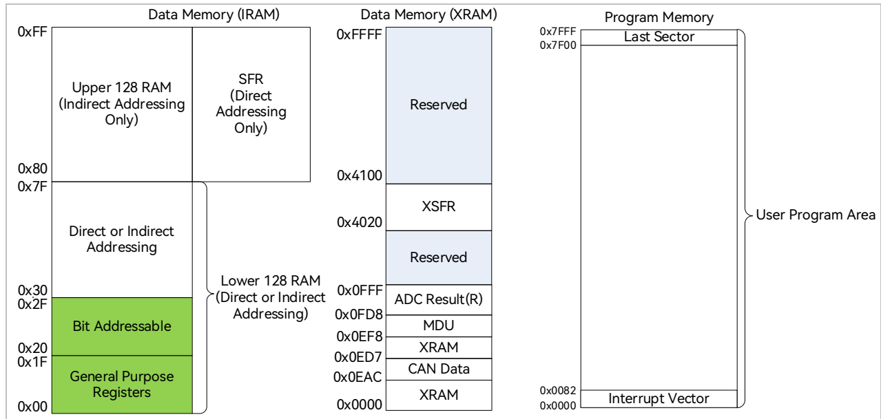
图 1-4 Memory 空间分配
