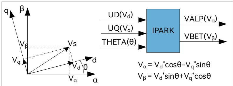
图 14-2 Park 逆变换
