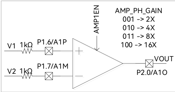
图 30-6 AMP1 工作在 PGA 差分输入模式
