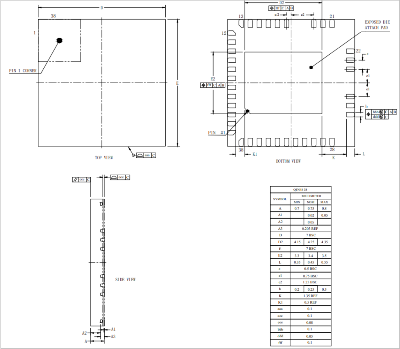
图 3-3 FU6867Q QFN48-38_7x7 封装尺寸图
