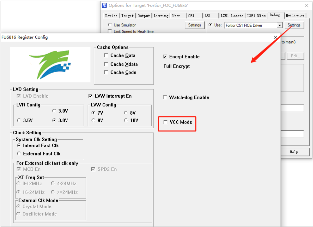
图 32-2 FU6816L VCC_MODE 配置
