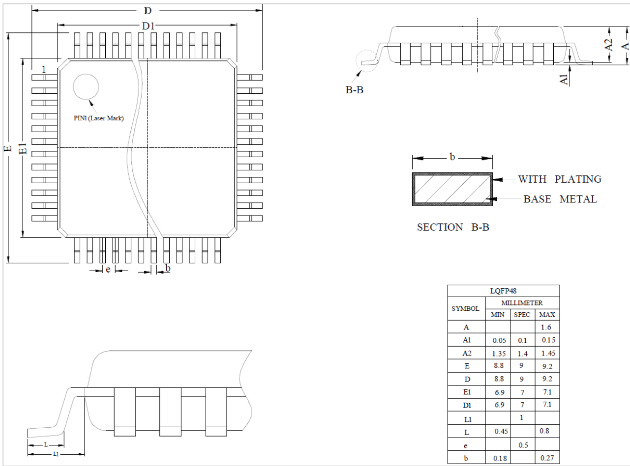
图 3-1 FU6816L LQFP48_7X7 封装尺寸图
