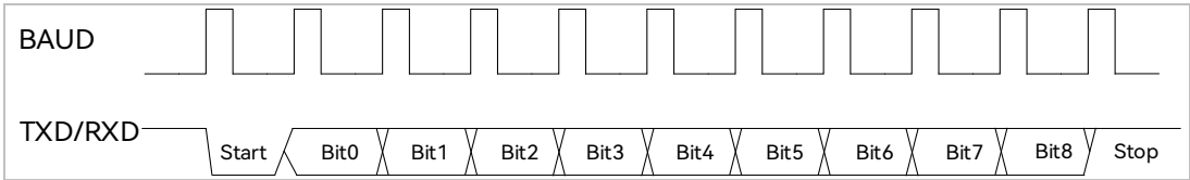
图 10-2 UART 通信时序图
