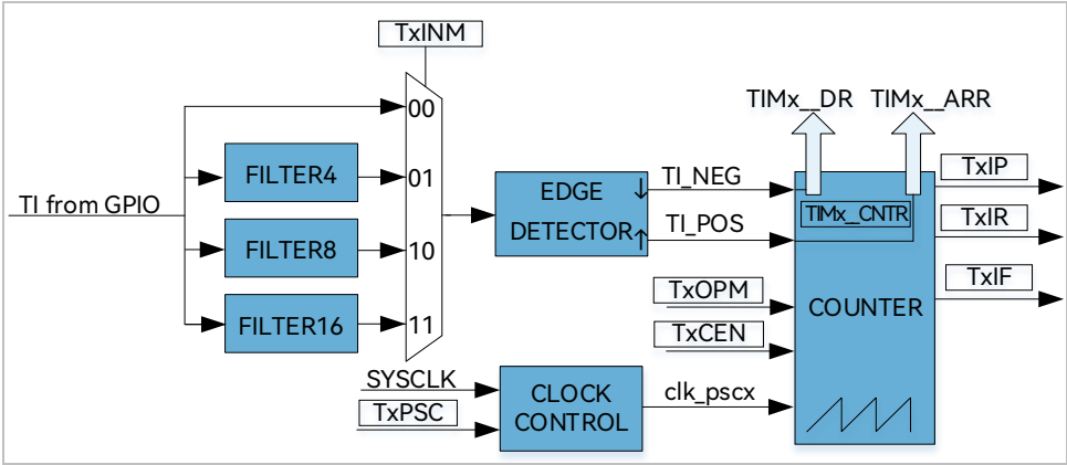
图 17-5 输入捕获模式原理框图
