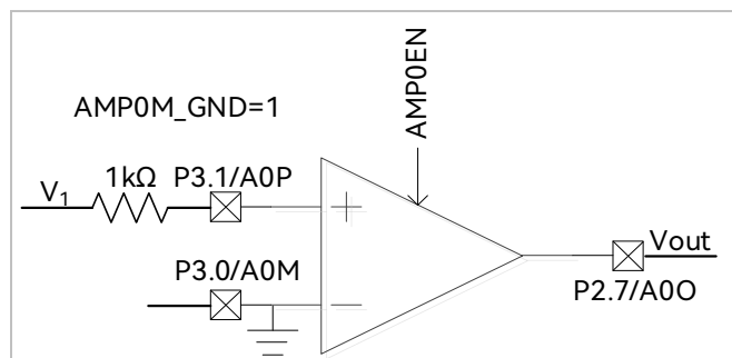
图 30-4 AMP0 工作在 PGA 单端输入模式
