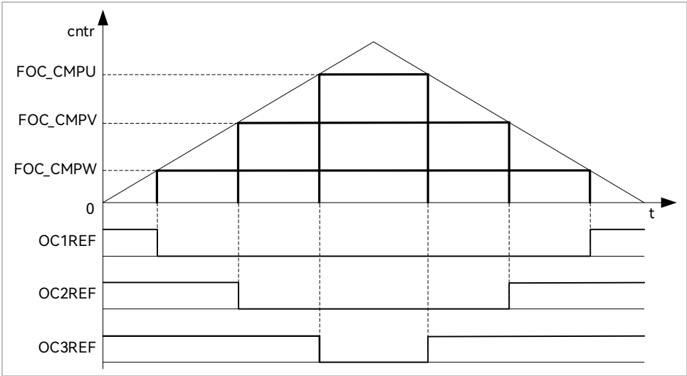
图 19-4 PWM 生成图
