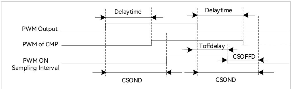
图 16-11 PWM ON 采样模式
