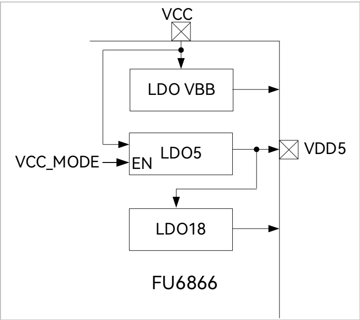
图 32-3 FU6866Q 电源模块功能框图
