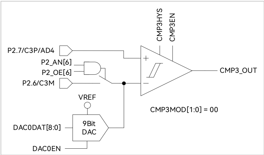
图 31-3 双比较器输入模式 (FU6867Q 不支持此模式)
