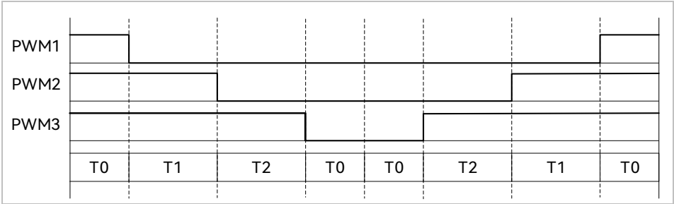
图 14-7 七段式 SVPWM 输出电平
