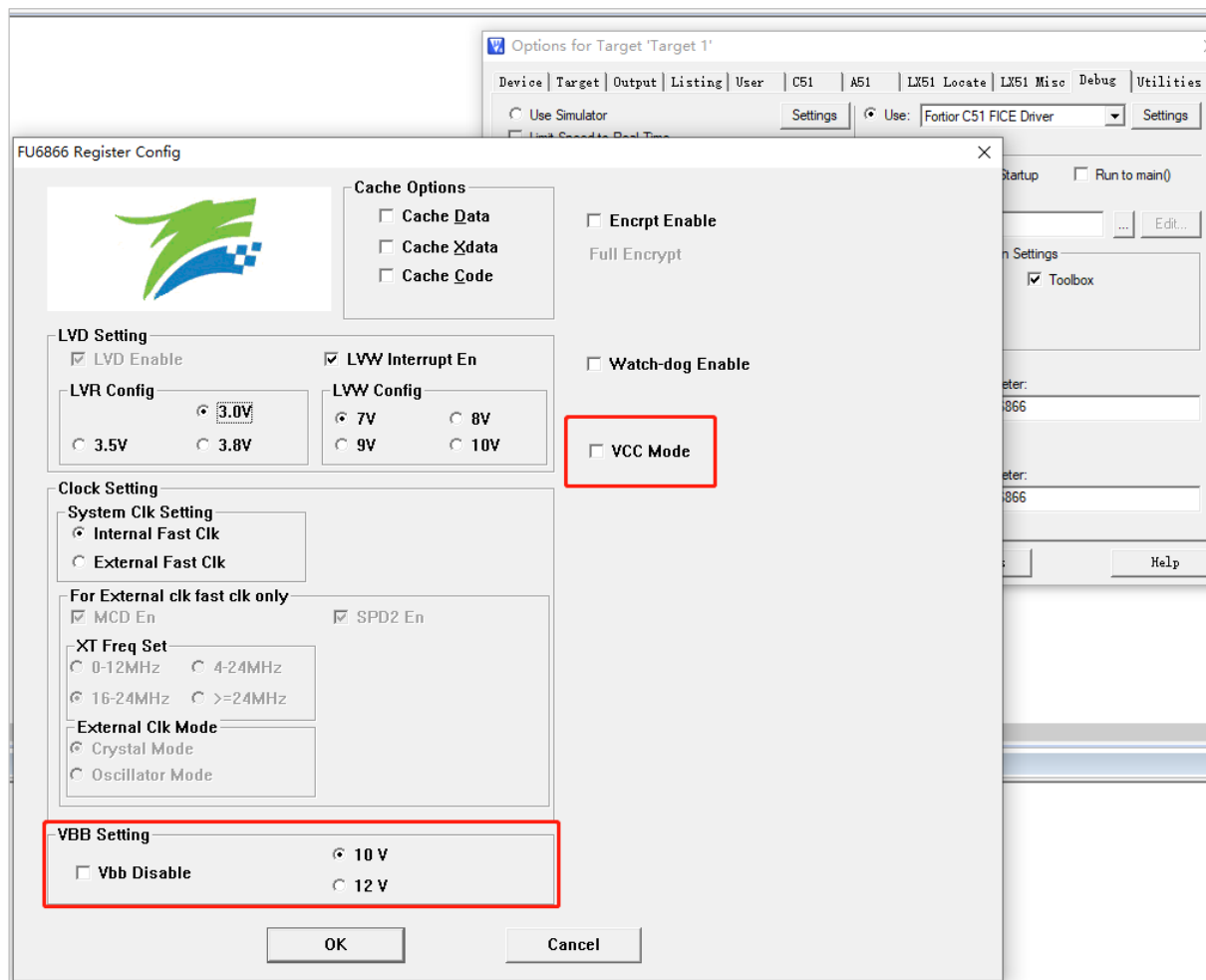
图 32-4 FU6866Q VCC_MODE 配置
