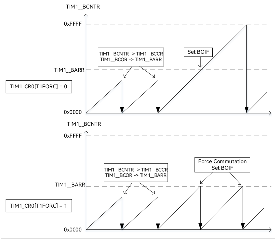
图 15-3 基本计数器计数波形图
