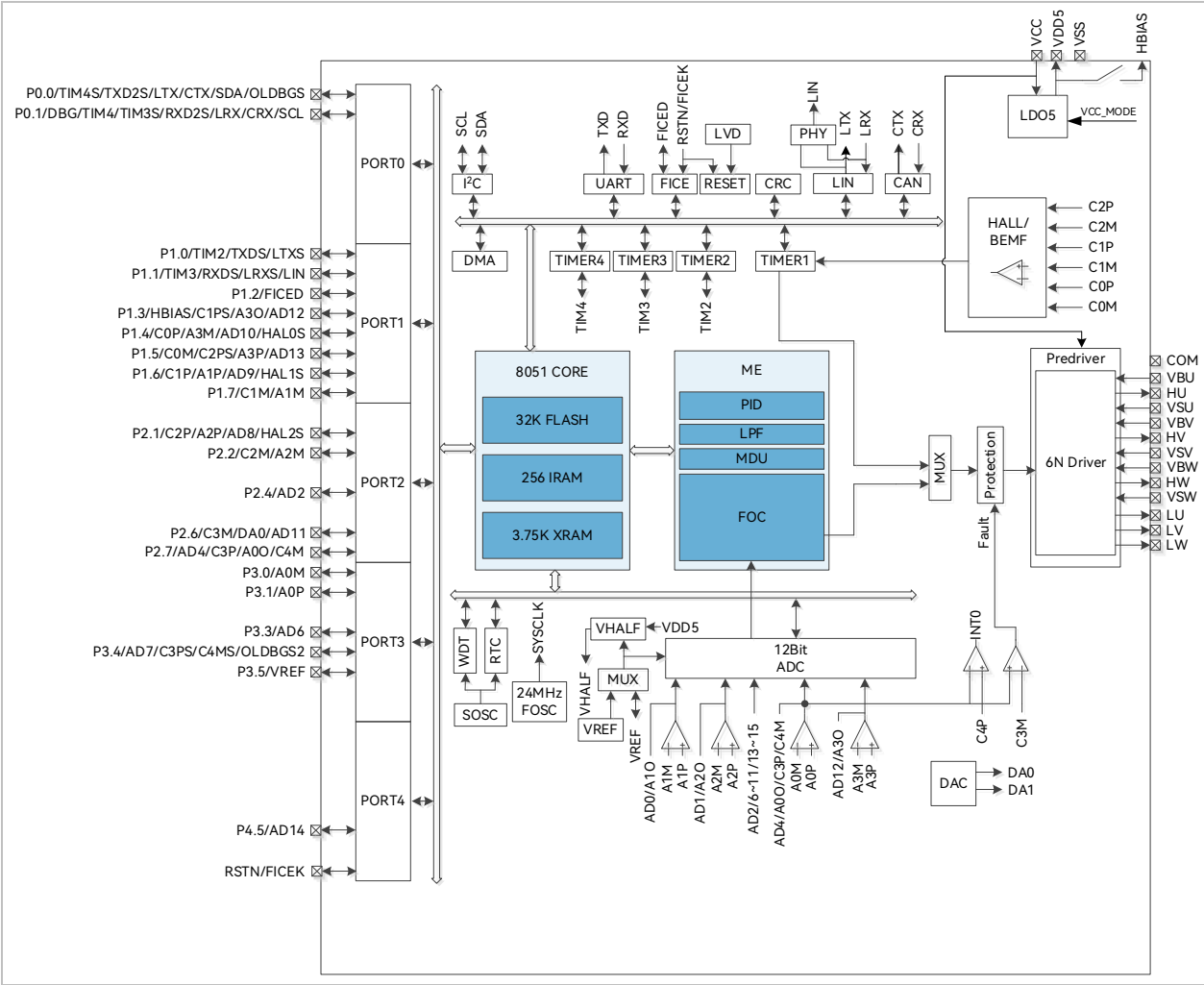
图 1-3 FU6867Q 功能框图
