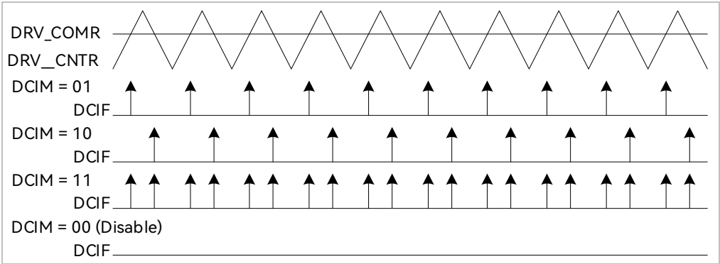
图 19-9 Driver 比较匹配中断
