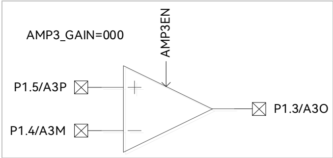
图 30-11 AMP3 输入输出相关端口
