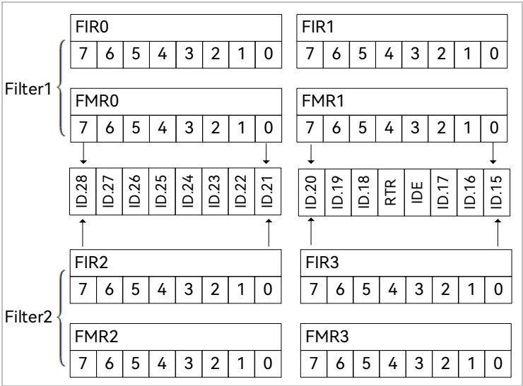
图 12-8 扩展帧双过滤器模式
