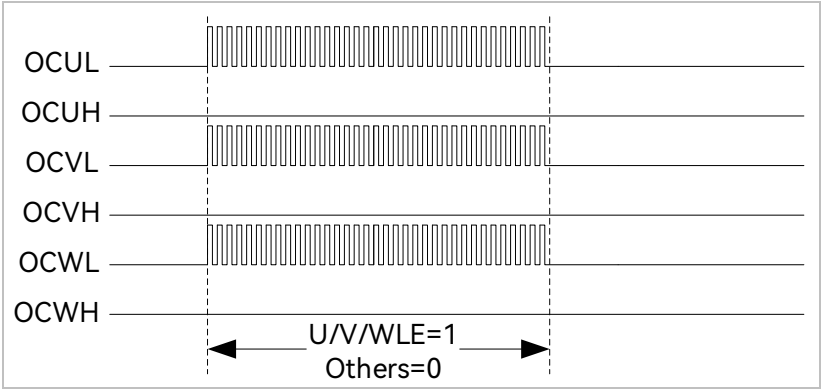
图 19-8 Timer1 自动控制 DRV_CM[R 和 CMP_CR2[4:3]
