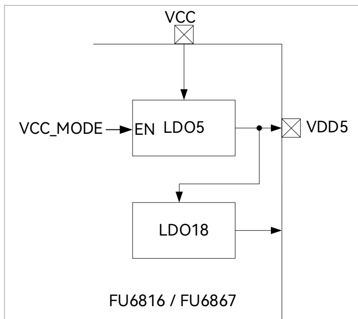
图 32-1 FU6816L/ FU6867Q 电源模块功能框图
