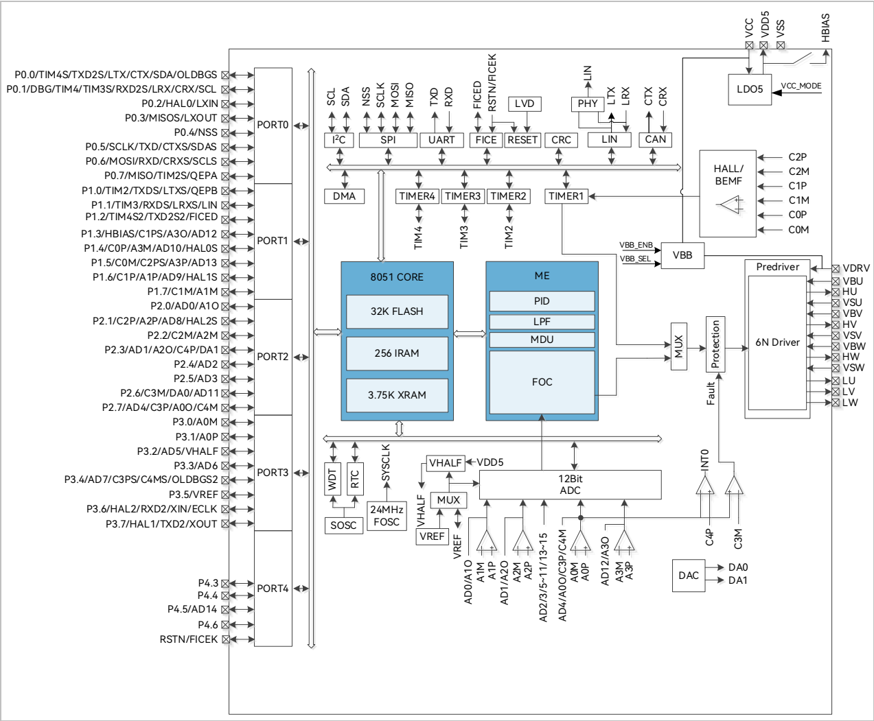
图 1-2 FU6866Q 功能框图
