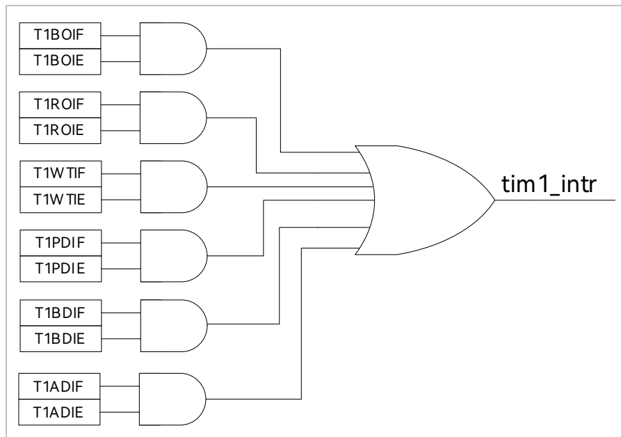
图 15-10 Timer1 中断源
