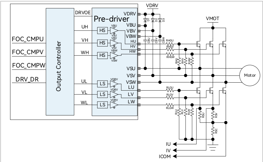
图 19-2 FU6867Q / FU6866Q Driver 模块框图
