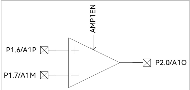
图 30-5 AMP1 输入输出相关端口
