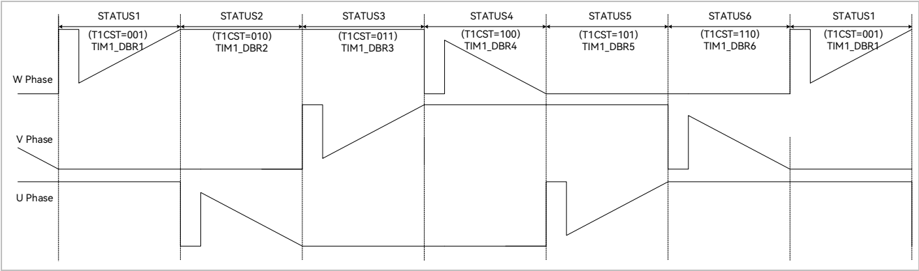
图 15-11 方波的六步换相图
