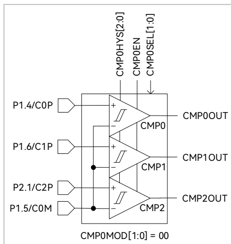
图 31-8 无内置电阻三比较器模式
