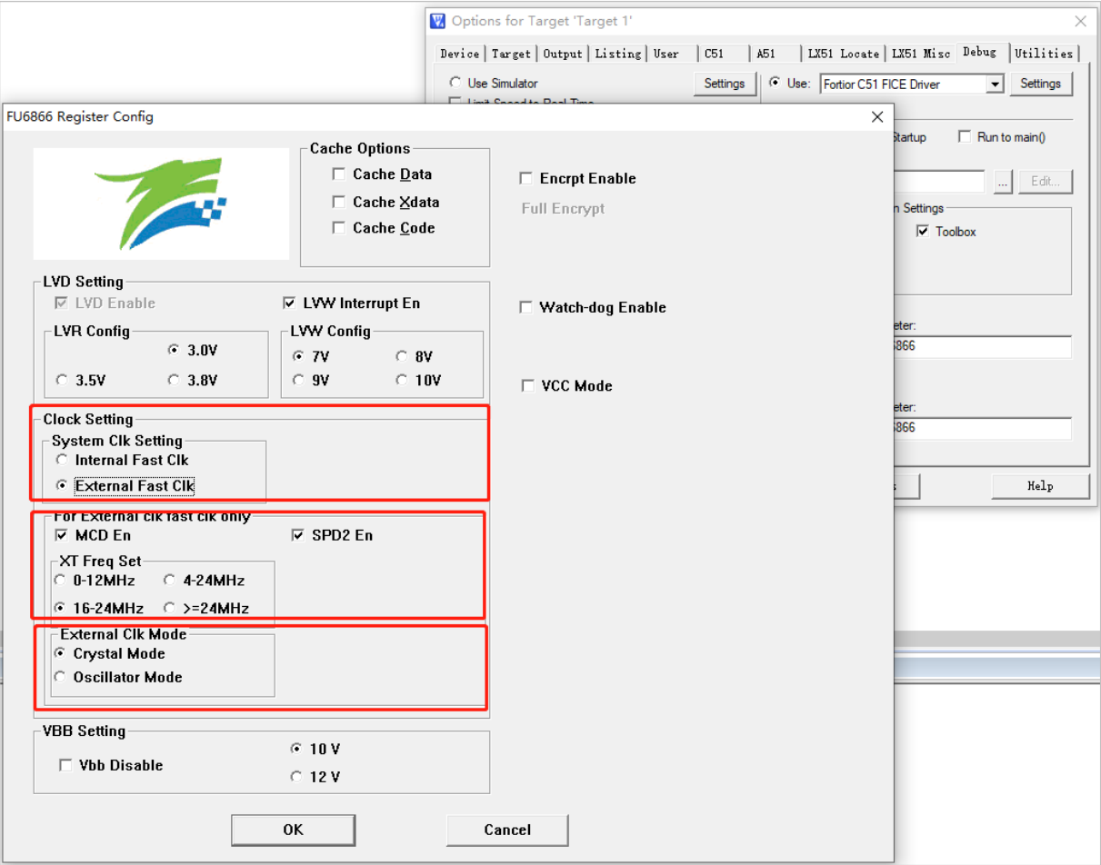
图 23-7 FU6866Q 系统时钟配置
