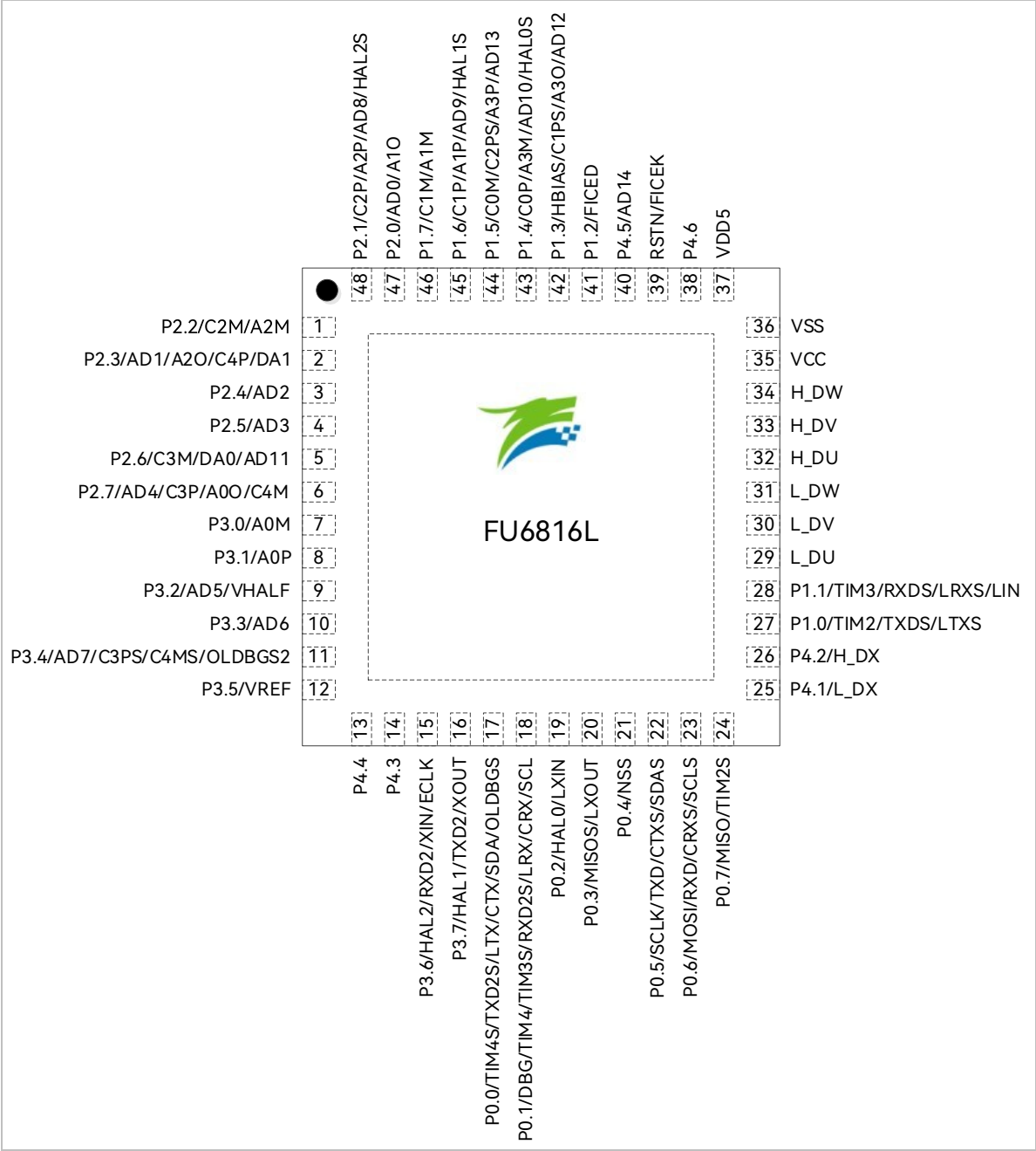
图 2-1 FU6816L LQFP48 引脚图
