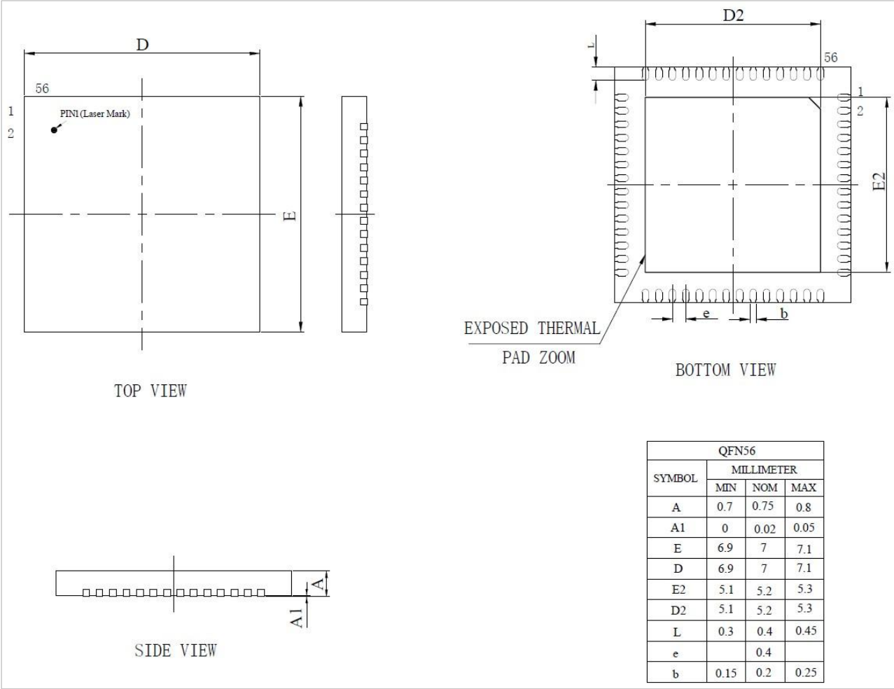
图 3-2 FU6866Q QFN56_7X7 封装尺寸图
