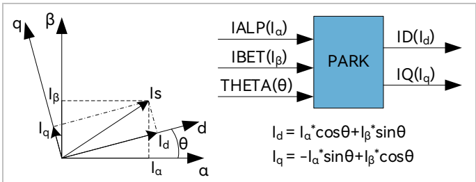
图 14-4 Park 变换
