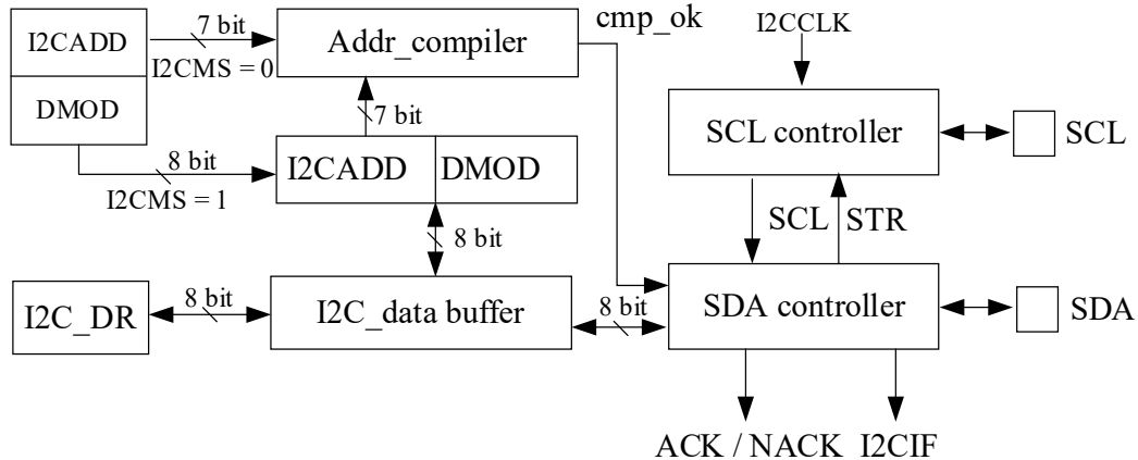
图 9-1 I 2 C 结构框图
