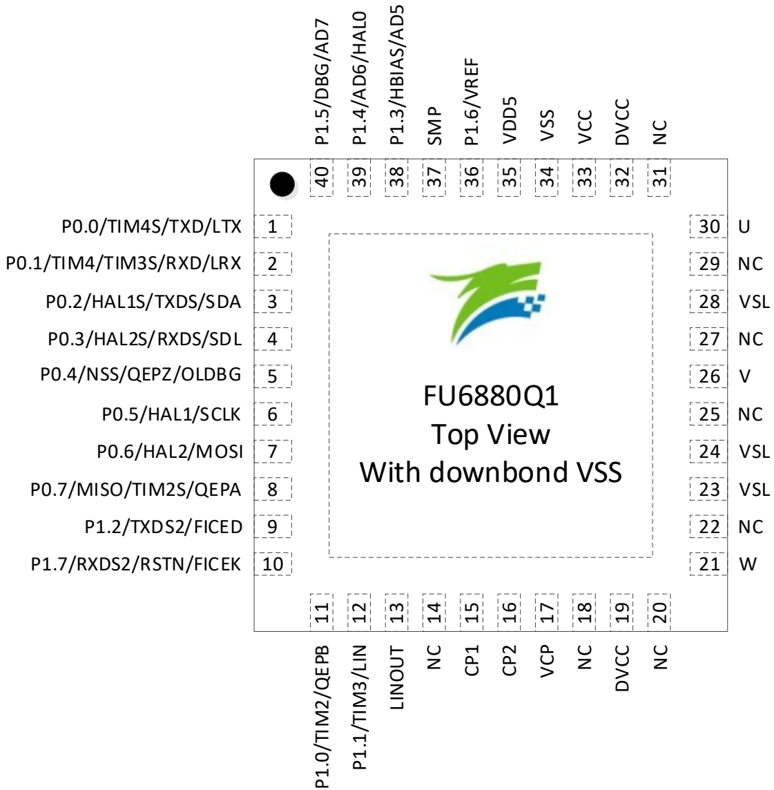
图 2-1 FU6880Q1 QFN40 引脚图
