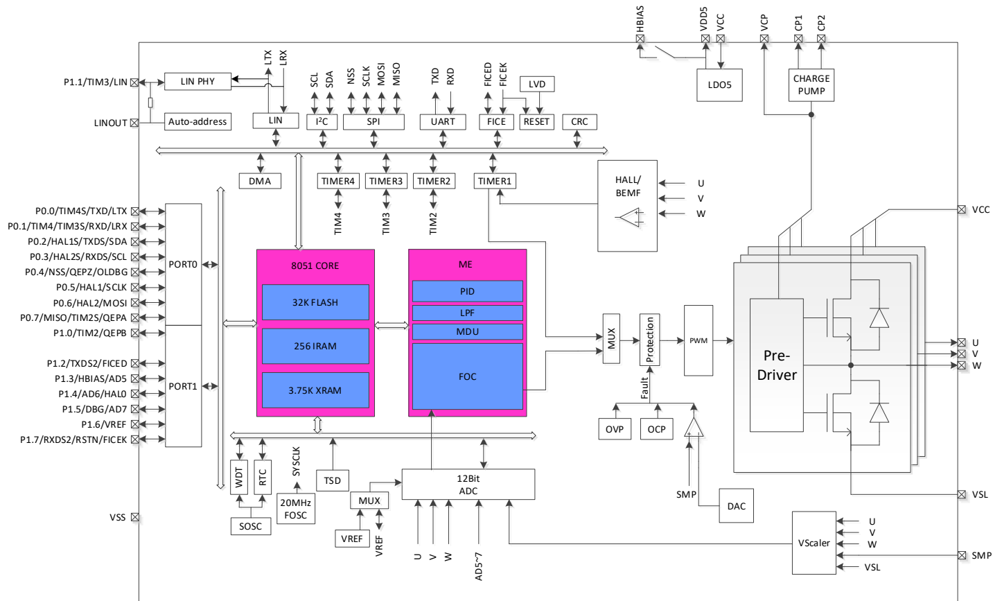
图 1-1 FU6880Q1 功能框图
