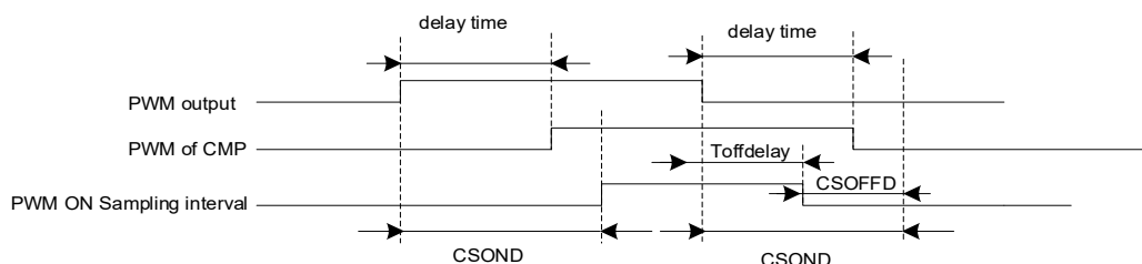
图 30-6 PWM ON 采样模式
