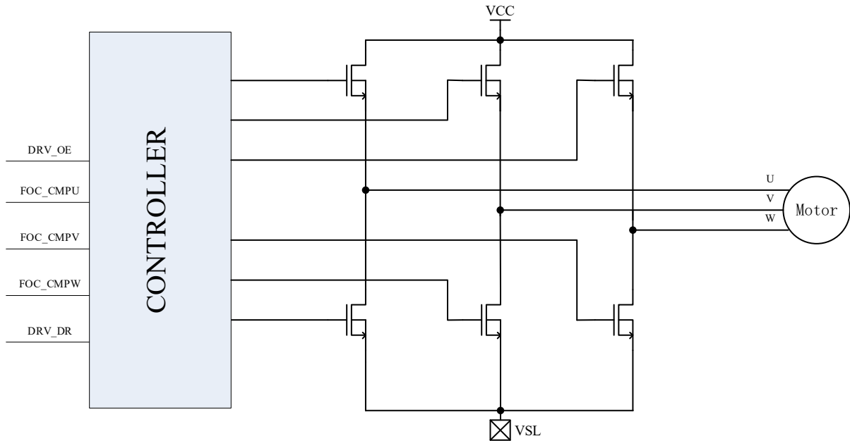
图 20-1 FU6880Q1 Driver 模块框图
