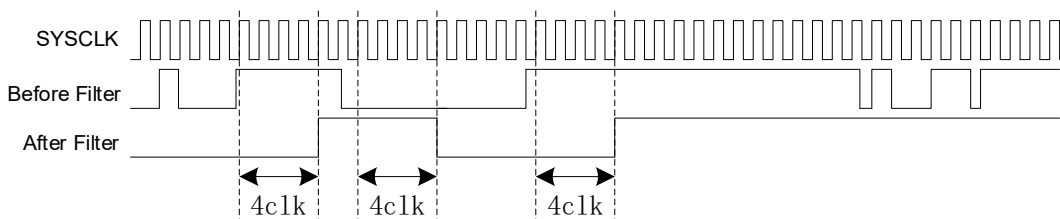
图 18-4 滤波模块时序图
