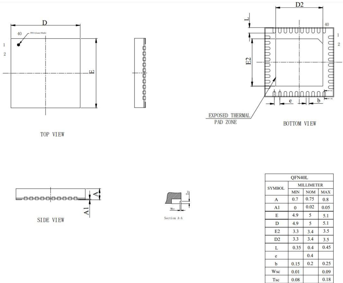
图 3-1 FU6880Q1 QFN40_5X5 封装尺寸图
