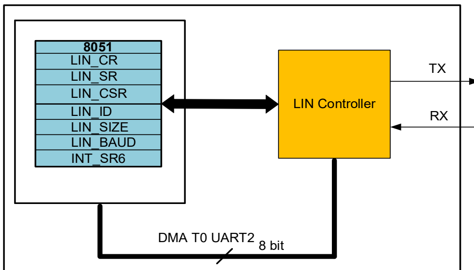
图 12-1 LIN 框图
