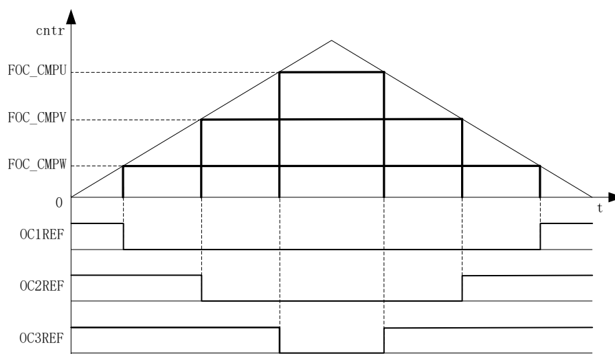
图 20-3 PWM 生成图
