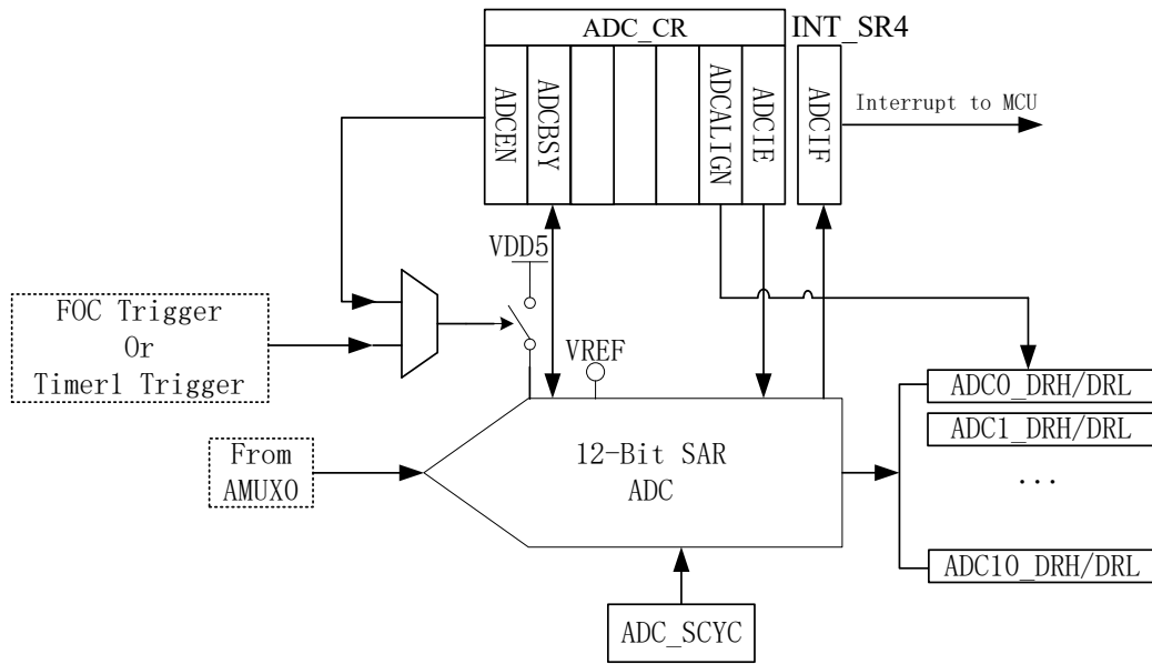
图 26-2 ADC 功能框图
