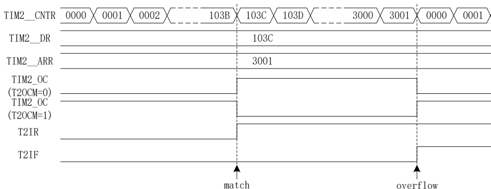
图 17-2 输出模式输出波形
