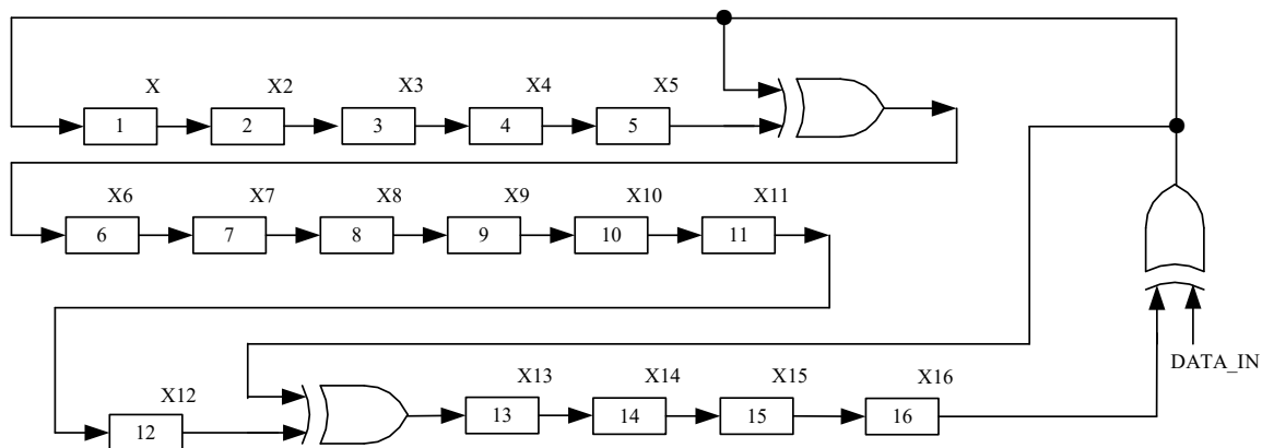
图 34-2 CRC16 电路原理图
